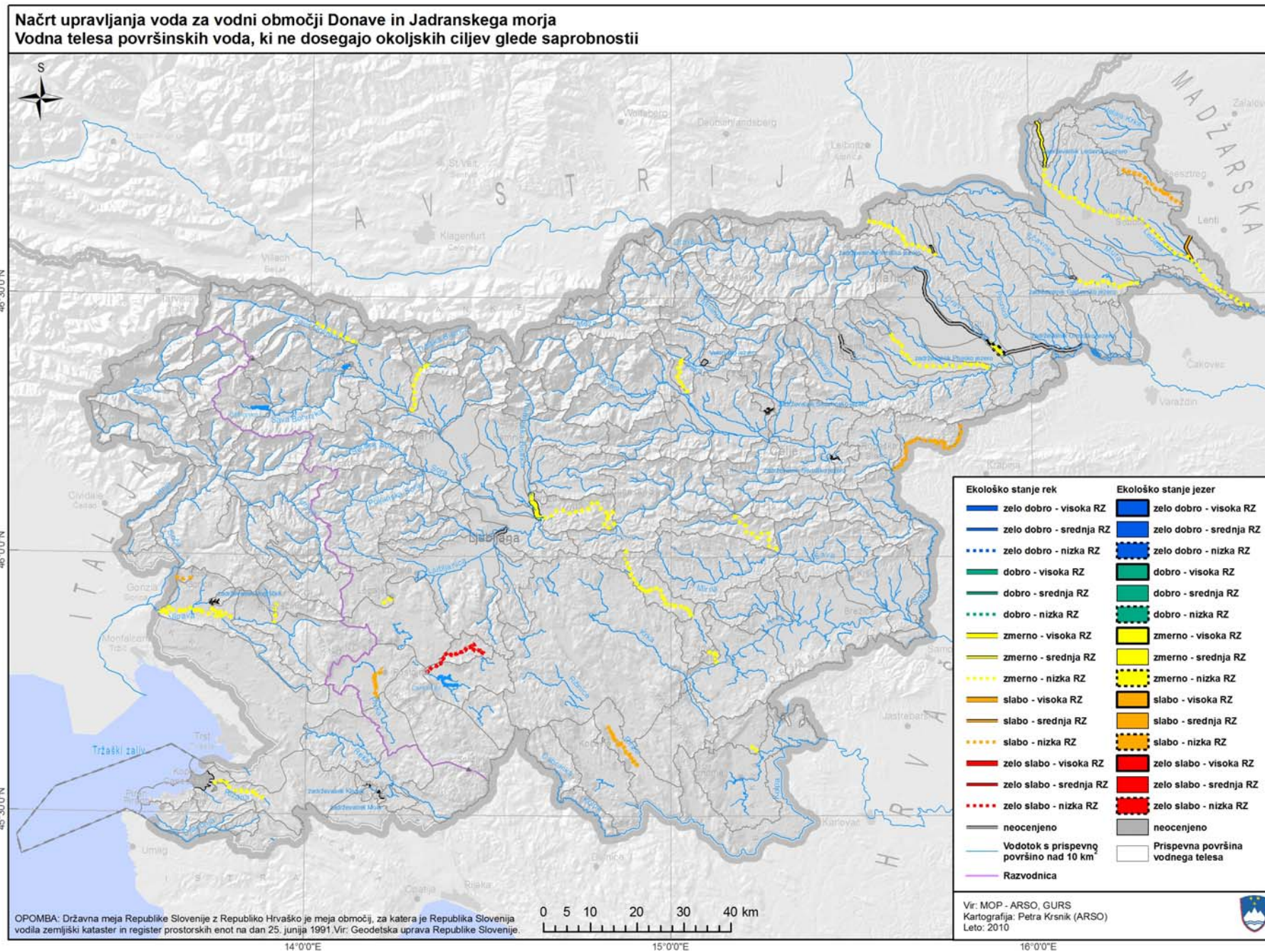
Karta 8: Vodna telesa površinskih voda, ki ne dosegajo okoljskih ciljev glede saprobnosti
