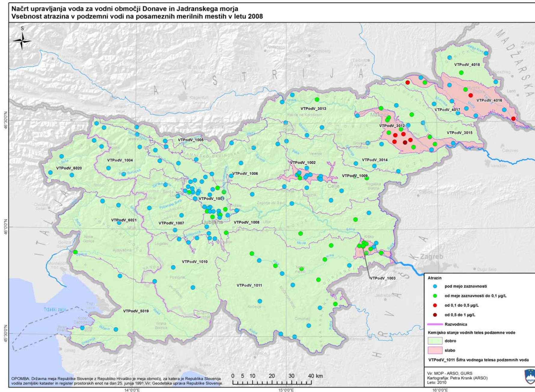
Karta 24: Vsebnost atrazina v podzemni vodi v letu 2008
