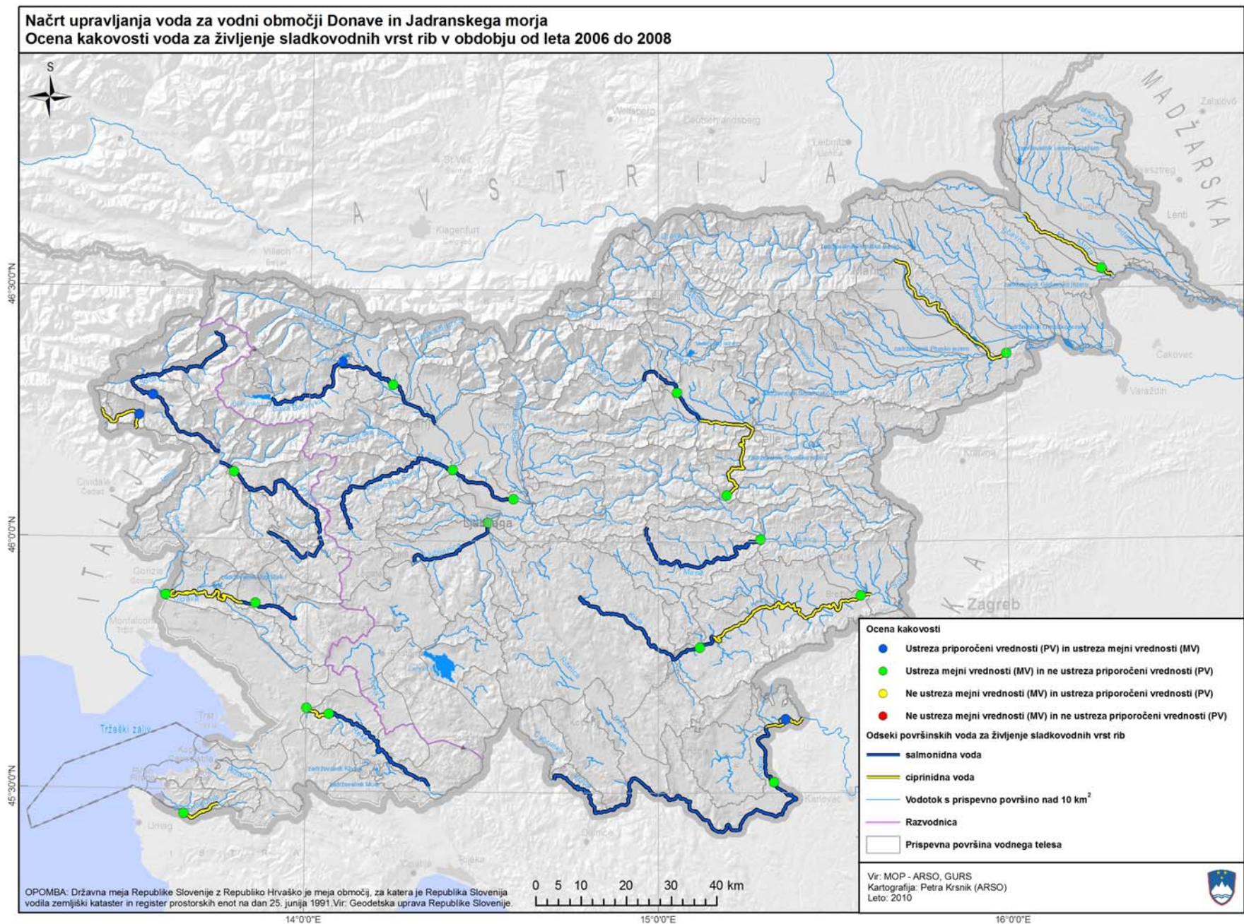
Karta 15: Kakovost vode za življenje sladkovodnih vrst rib v obdobju 2006 do 2008
