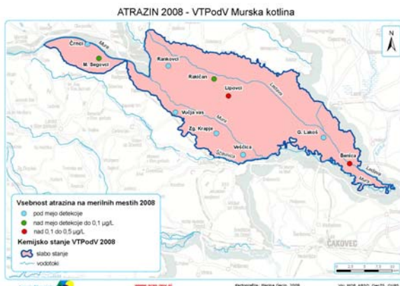
Slika 27: Vsebnost atrazina na merilnih mestih vodnega telesa podzemne vode Murska kotlina v letu 2008
