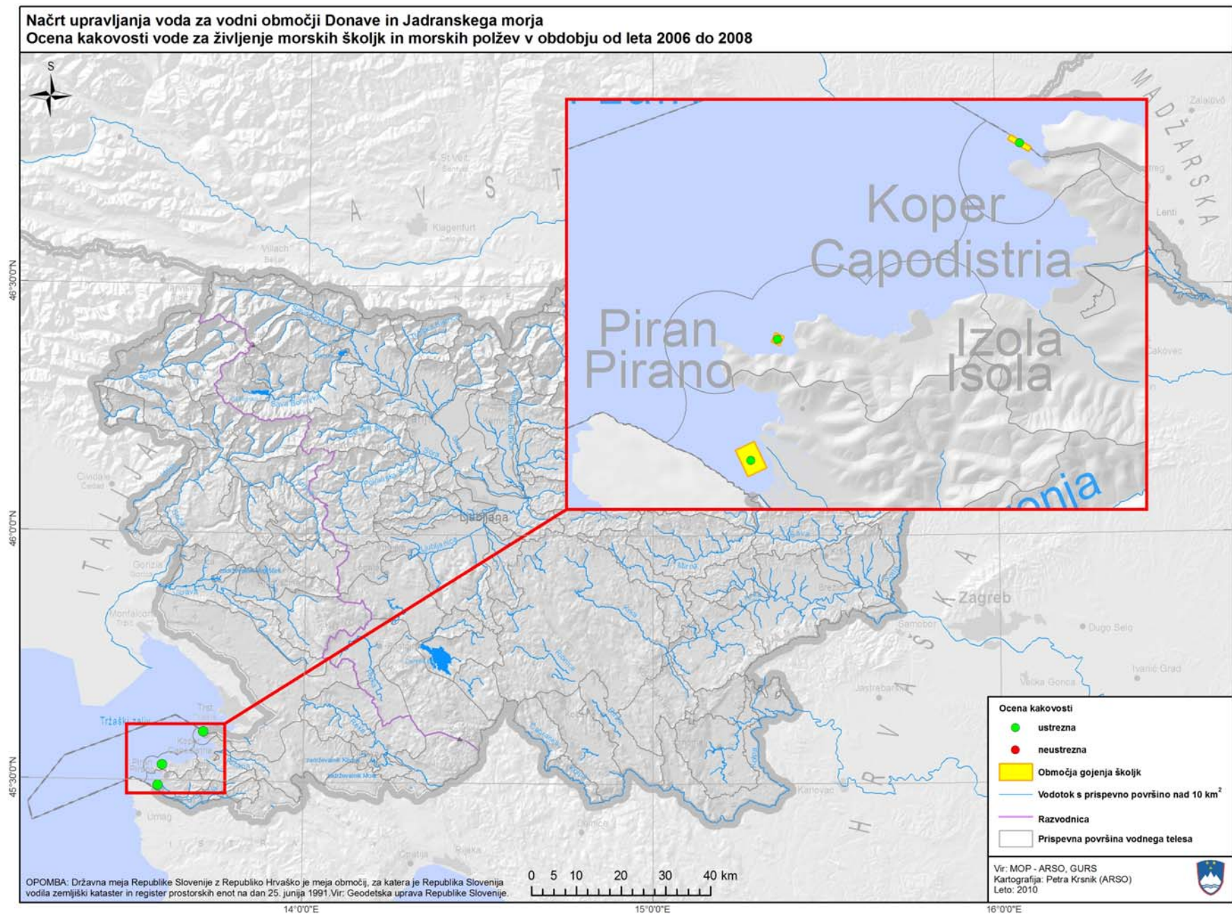
Karta 16: Kakovost vode za življenje morskih školjk in morskih polžev
