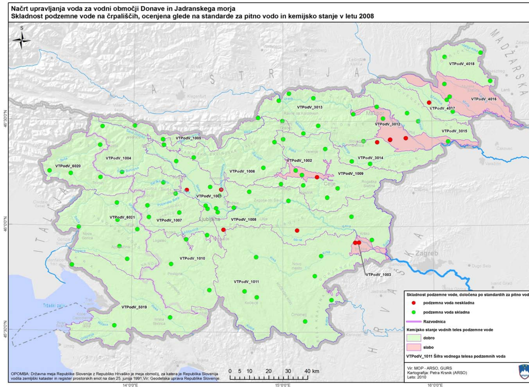
Karta 10: Črpališča, vključena v monitoring kemijskega stanja podzemne vode, kjer kakovost vode ne ustreza zahtevam za pitno vodo
