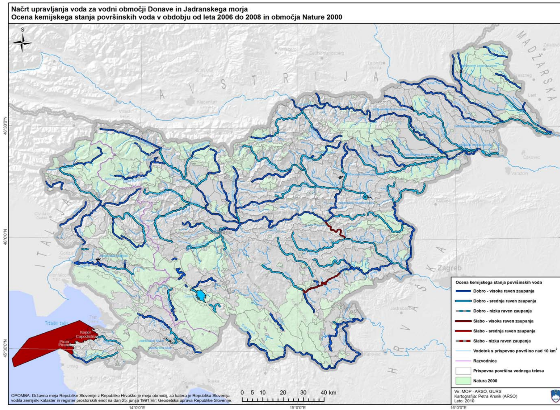
Karta 18: Ocena kemijskega stanja površinskih voda v obdobju od leta 2006 do 2008 in območja Nature 2000
