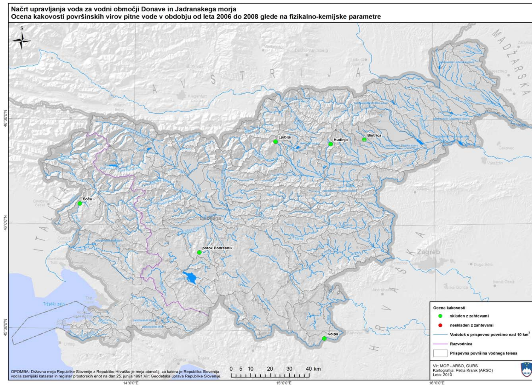
Karta 12: Ocena kakovosti površinskih voda, ki se jih odvzema za oskrbo s pitno vodo v obdobju 2006 do 2008 glede na fizikalno-kemijske parametre
