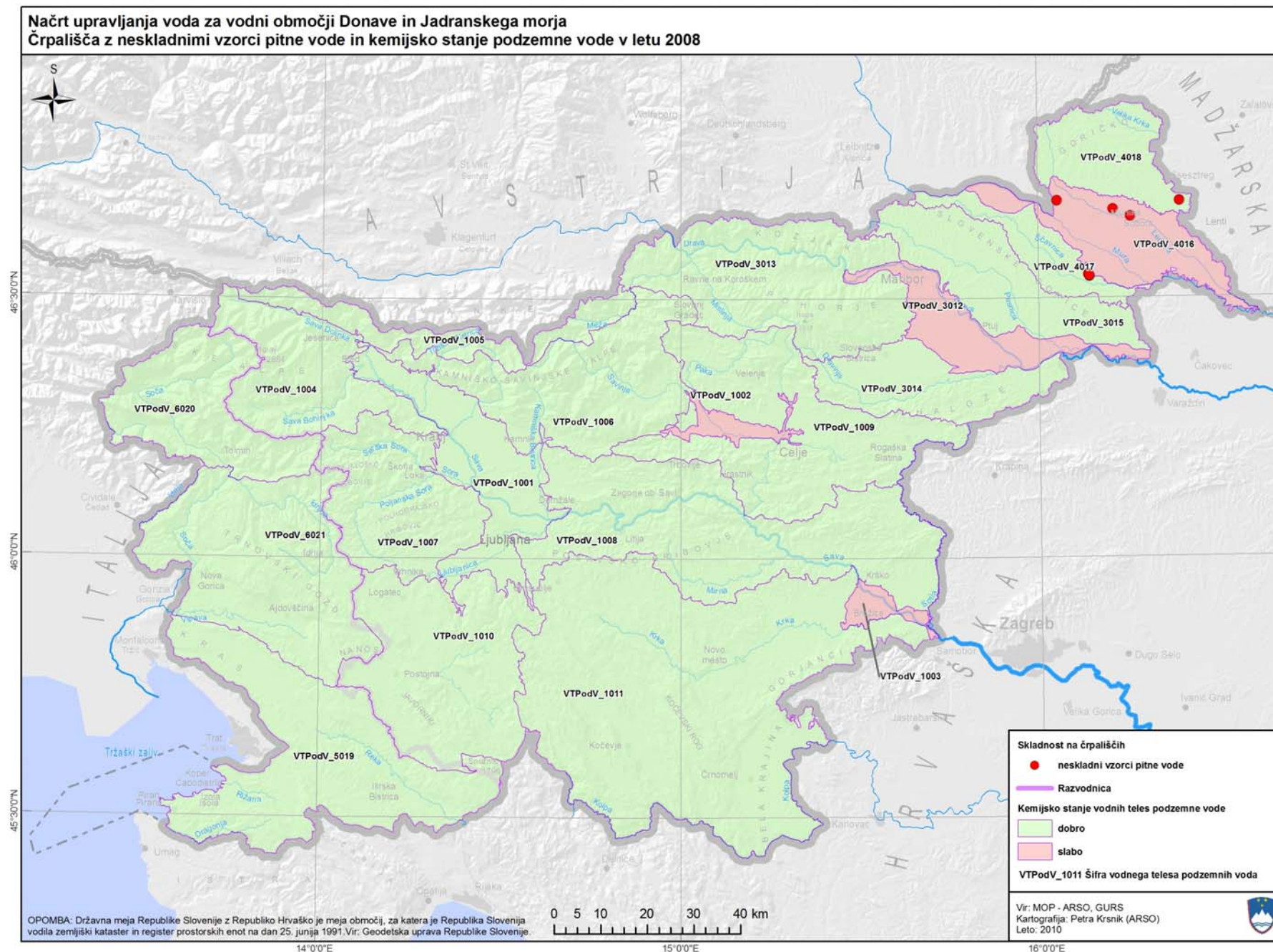
Karta 11: Črpališča z neskladnimi vzorci pitne vode glede fizikalno-kemijskih parametrov v letu 2008
