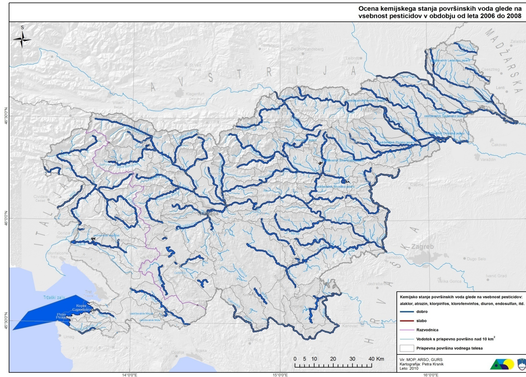
Karta 4: Vodna telesa površinskih voda, ki ne dosegajo okoljskih ciljev zaradi preseganja standarda kakovosti za pesticide iz prednostne liste
