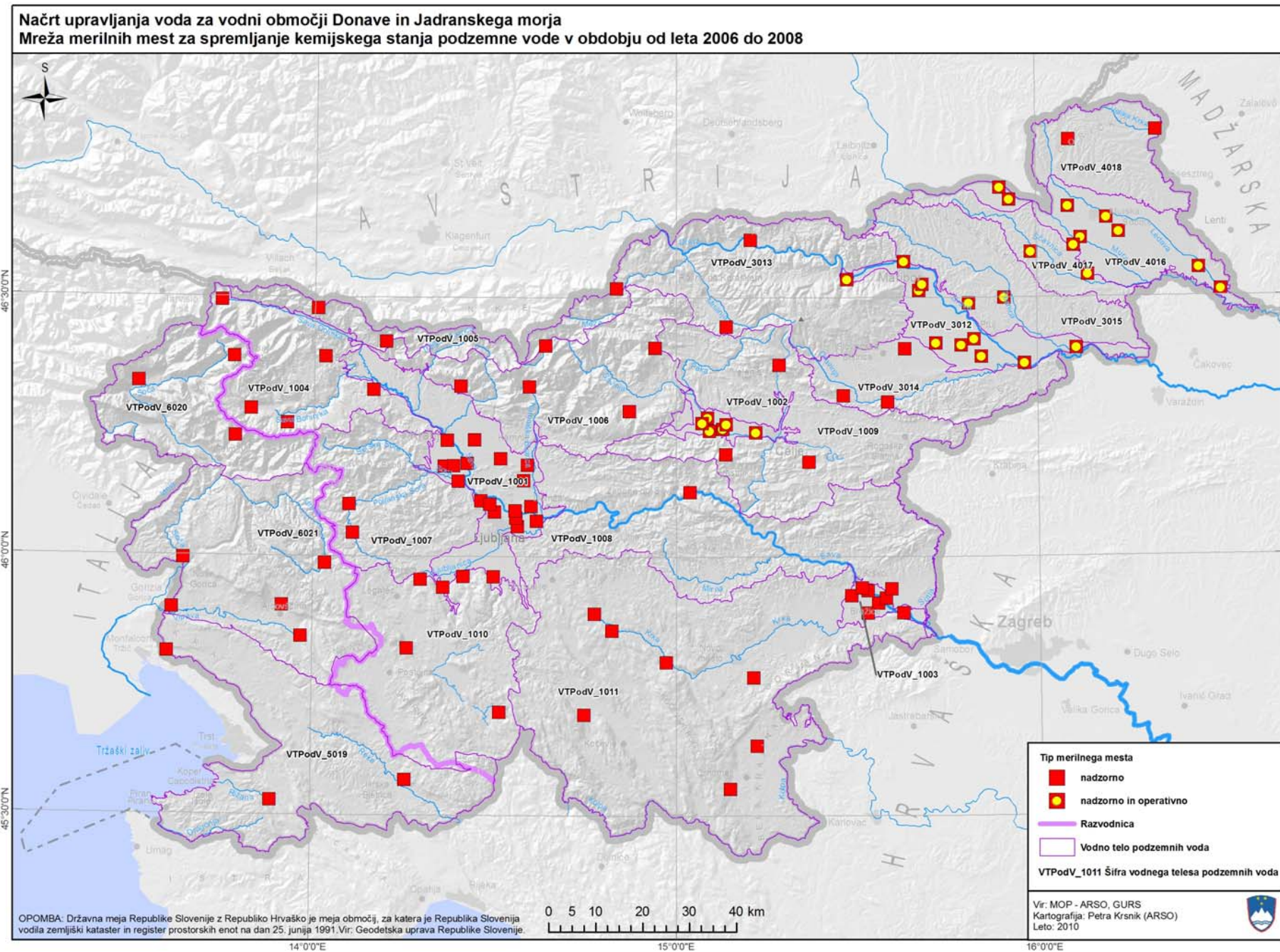
Karta 20: Mreža merilnih mest za spremljanje kemijskega stanja podzemne vode
