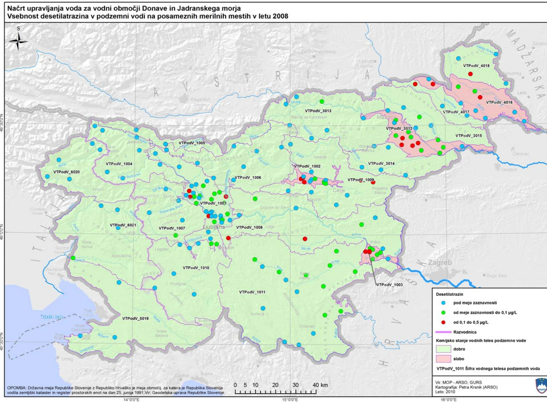
Karta 25: Vsebnost desetil-atrazina v podzemni vodi v letu 2008
