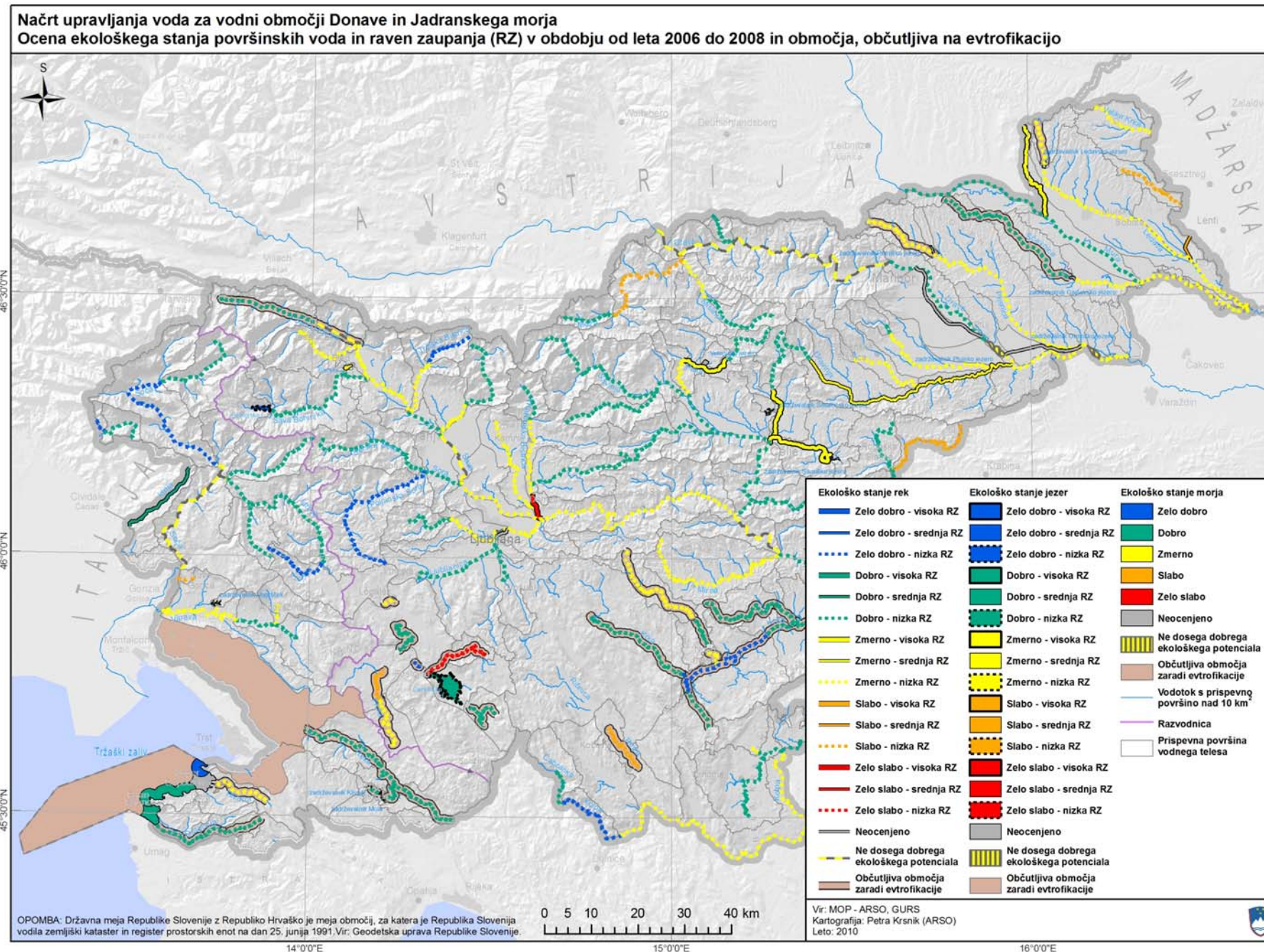
Karta 17: Ekološko stanje površinskih voda in območja, občutljiva na eutrofikacijo
