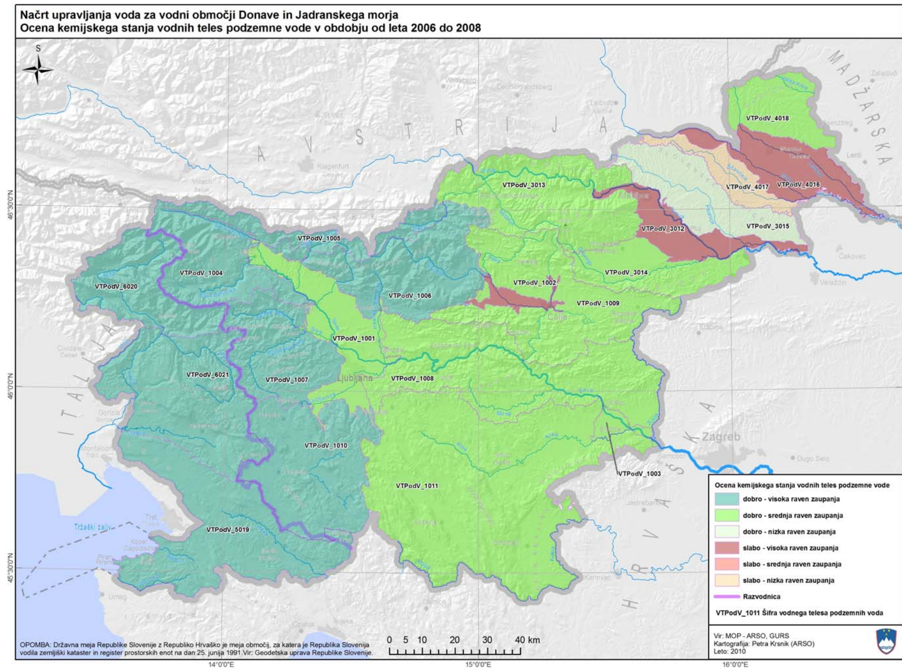
Karta 21: Ocena kemijskega stanja podzemne vode v obdobju od 2006 do 2008
