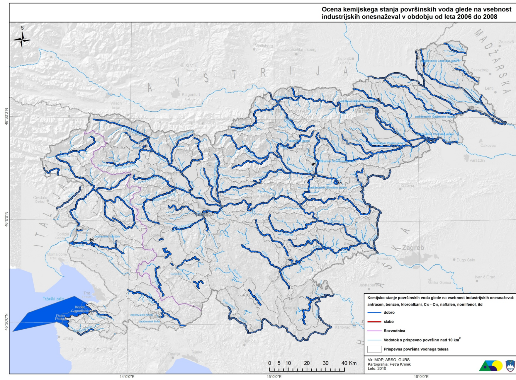
Karta 5: Vodna telesa površinskih voda, ki ne dosegajo okoljskih ciljev zaradi preseganja standarda kakovosti za industrijska onesnaževala iz prednostne liste
