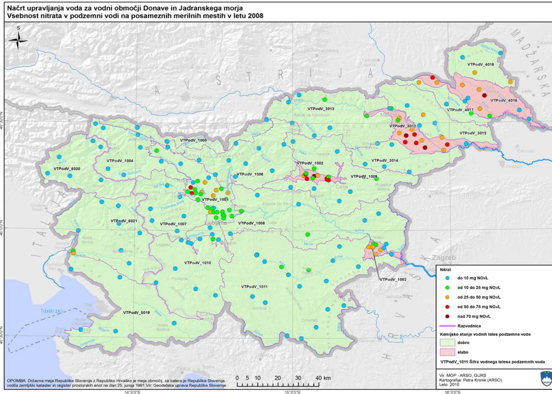
Karta 22: Vsebnost nitrata v podzemni vodi v letu 2008
