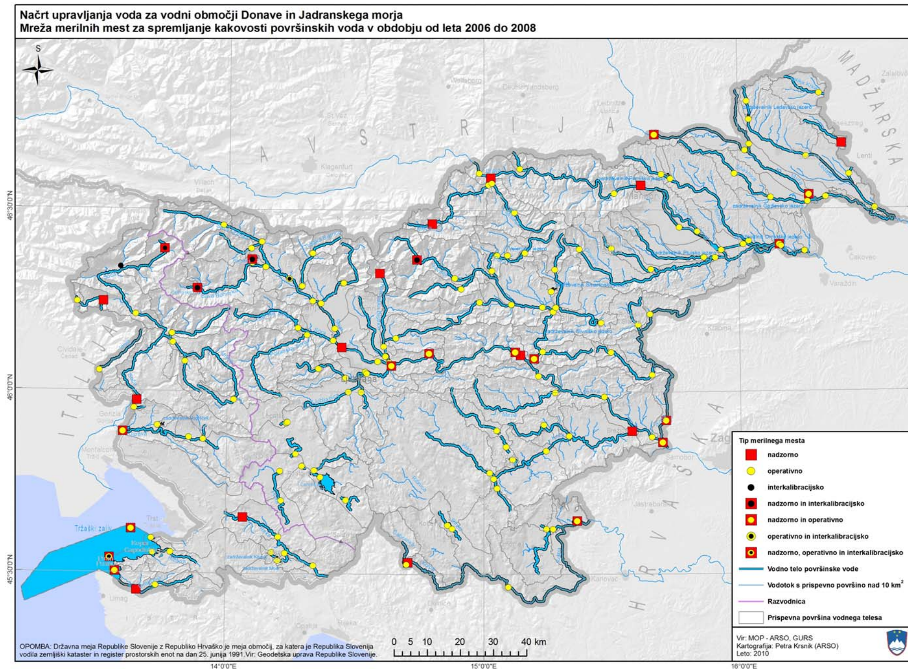
Karta 1: Mreža merilnih mest za spremljanje kakovosti površinskih voda v obdobju od 2006 do 2008
