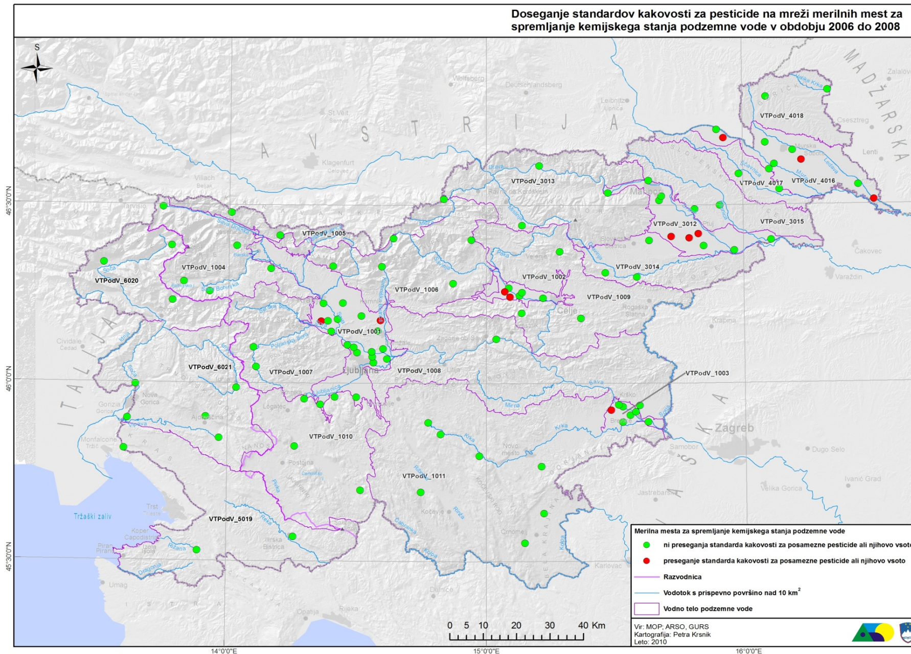
Karta 23: Obremenjenost podzemne vode s pesticidi
