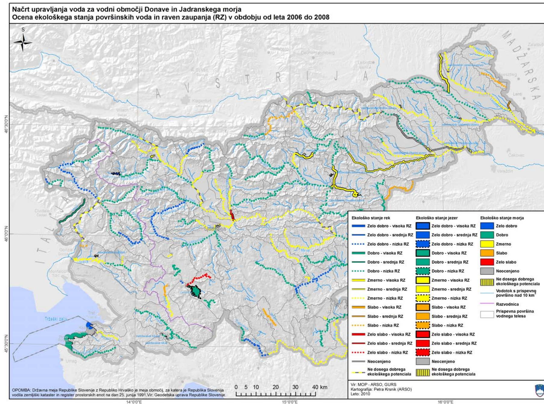
Karta 6: Ocena ekološkega stanja površinskih voda v obdobju od leta 2006 do 2008
