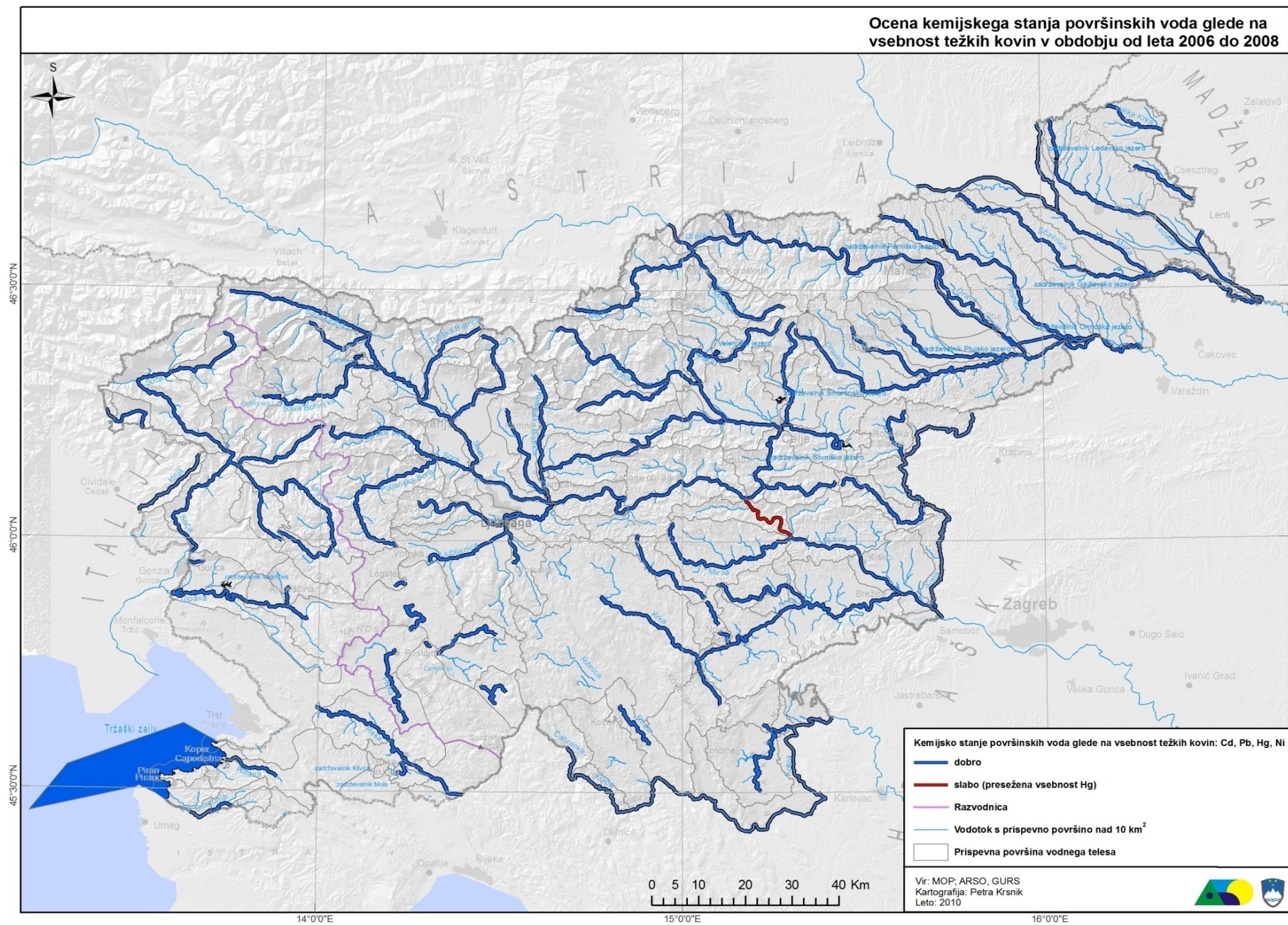
Karta 3: Vodna telesa površinskih voda, ki ne dosegajo okoljskih ciljev zaradi preseganja standarda kakovosti za težke kovine iz prednostne liste
