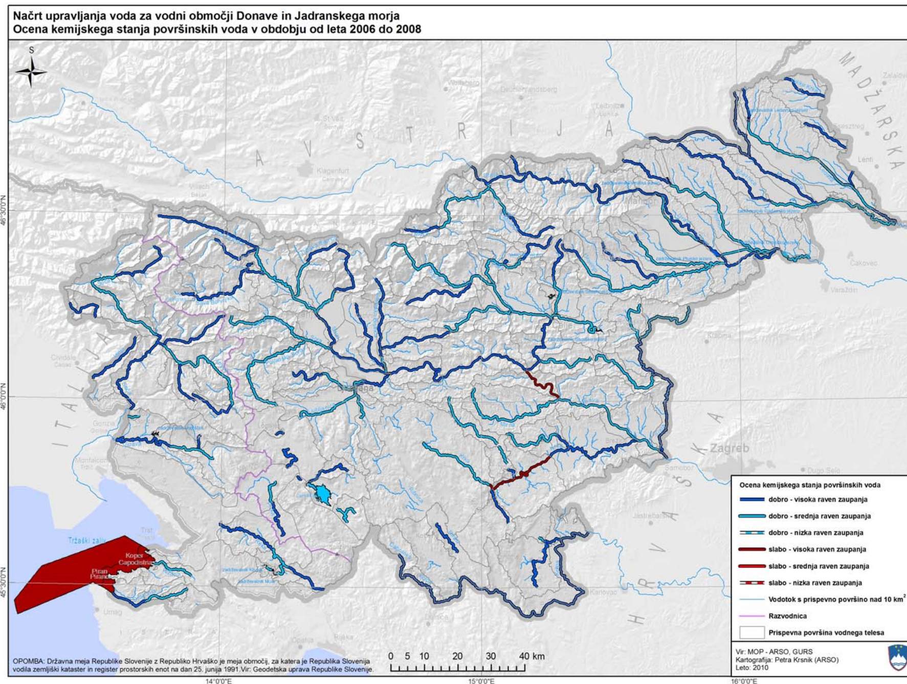
Karta 2: Ocena kemijskega stanja površinskih voda v obdobju od leta 2006 do 2008
