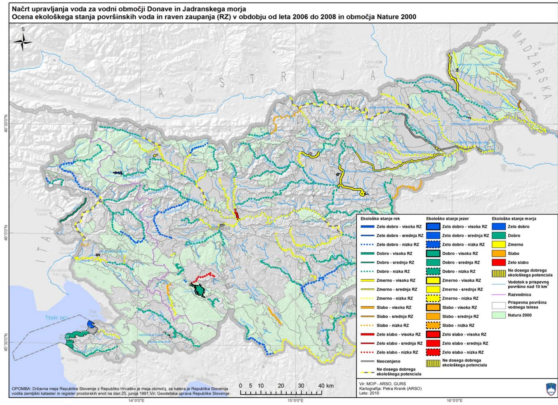
Karta 19: Ocena ekološkega stanja površinskih voda v obdobju od leta 2006 do 2008 in območja Nature 2000
