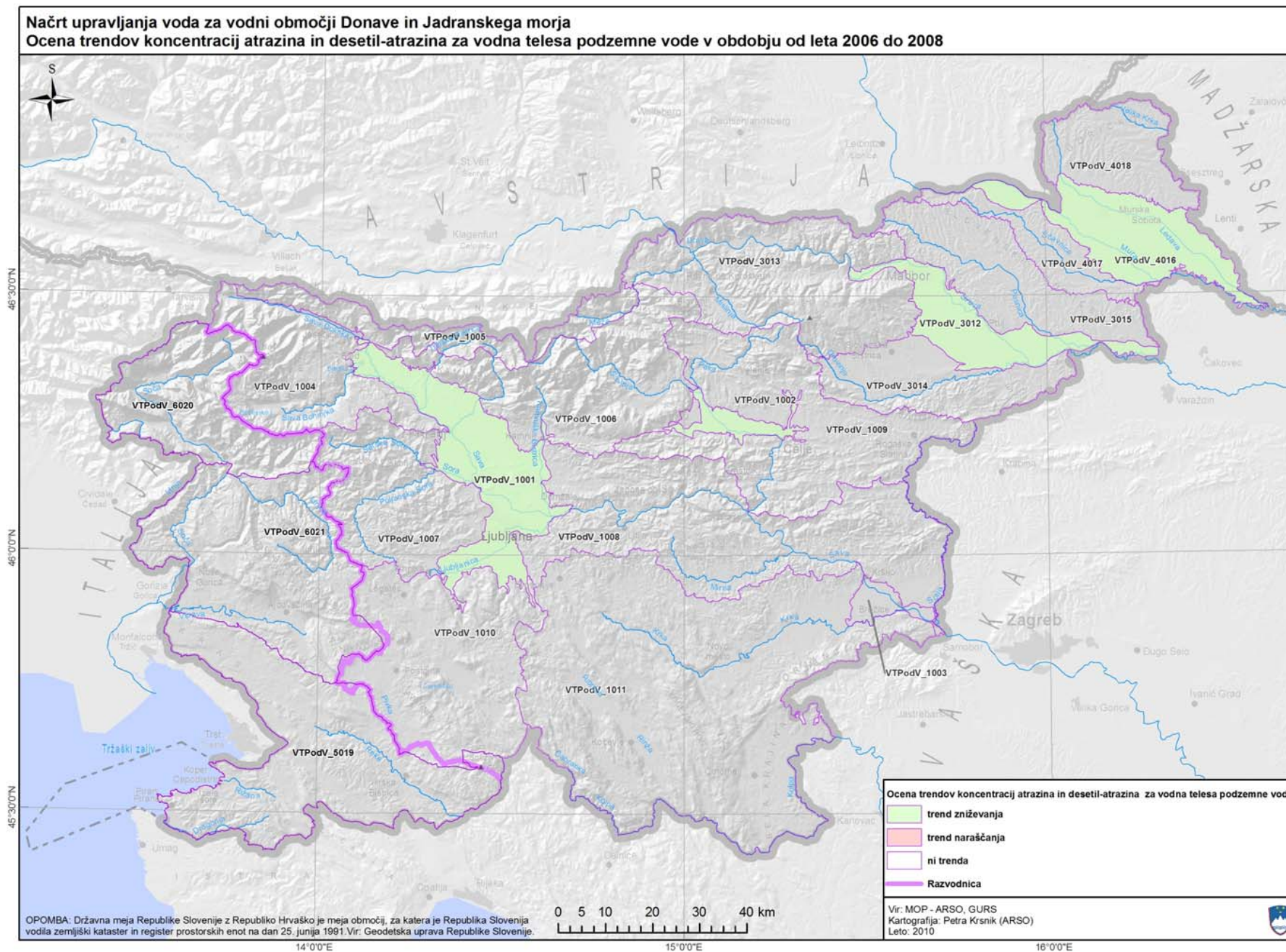
Karta 26: Trendi upadanja atrazina in desetil-atrazina v vodnih telesih podzemne vode
