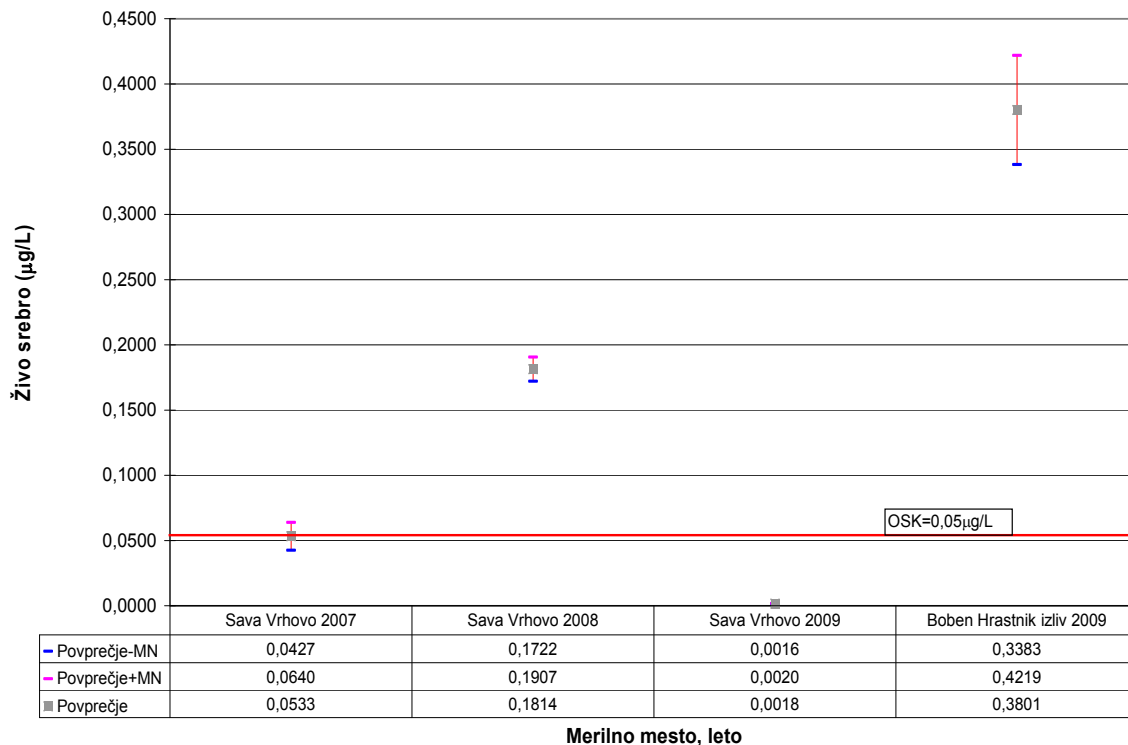
Slika 10: Povprečne letne vsebnosti živega srebra z upoštevanjem merilne negotovosti analitskih metod v vodnem telesu Sava Vrhovo Boštanj in v potoku Boben
