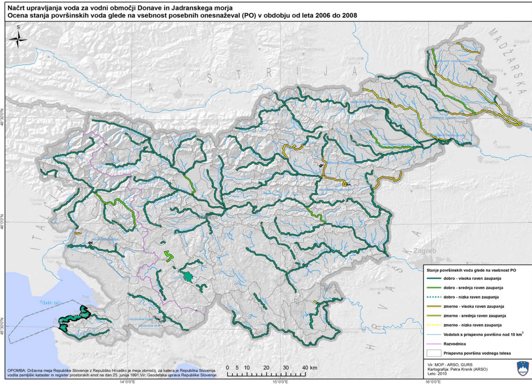
Karta 9: Vodna telesa površinskih voda, ki ne dosegajo okoljskih ciljev zaradi posebnih onesnaževal
