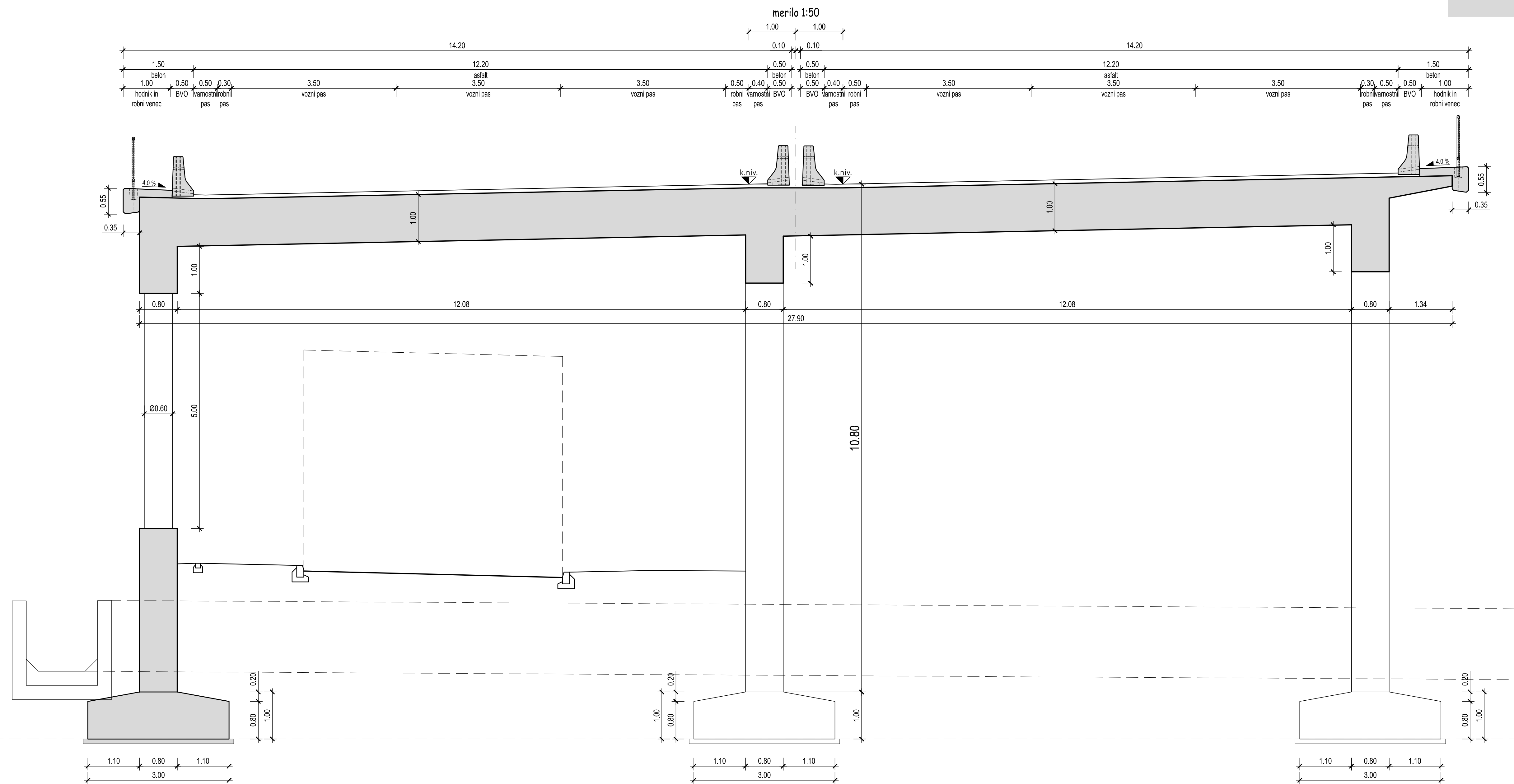
GALERIJA 8-05 PESJE KARAKTERISTIČNA PREČNA PREREZA
