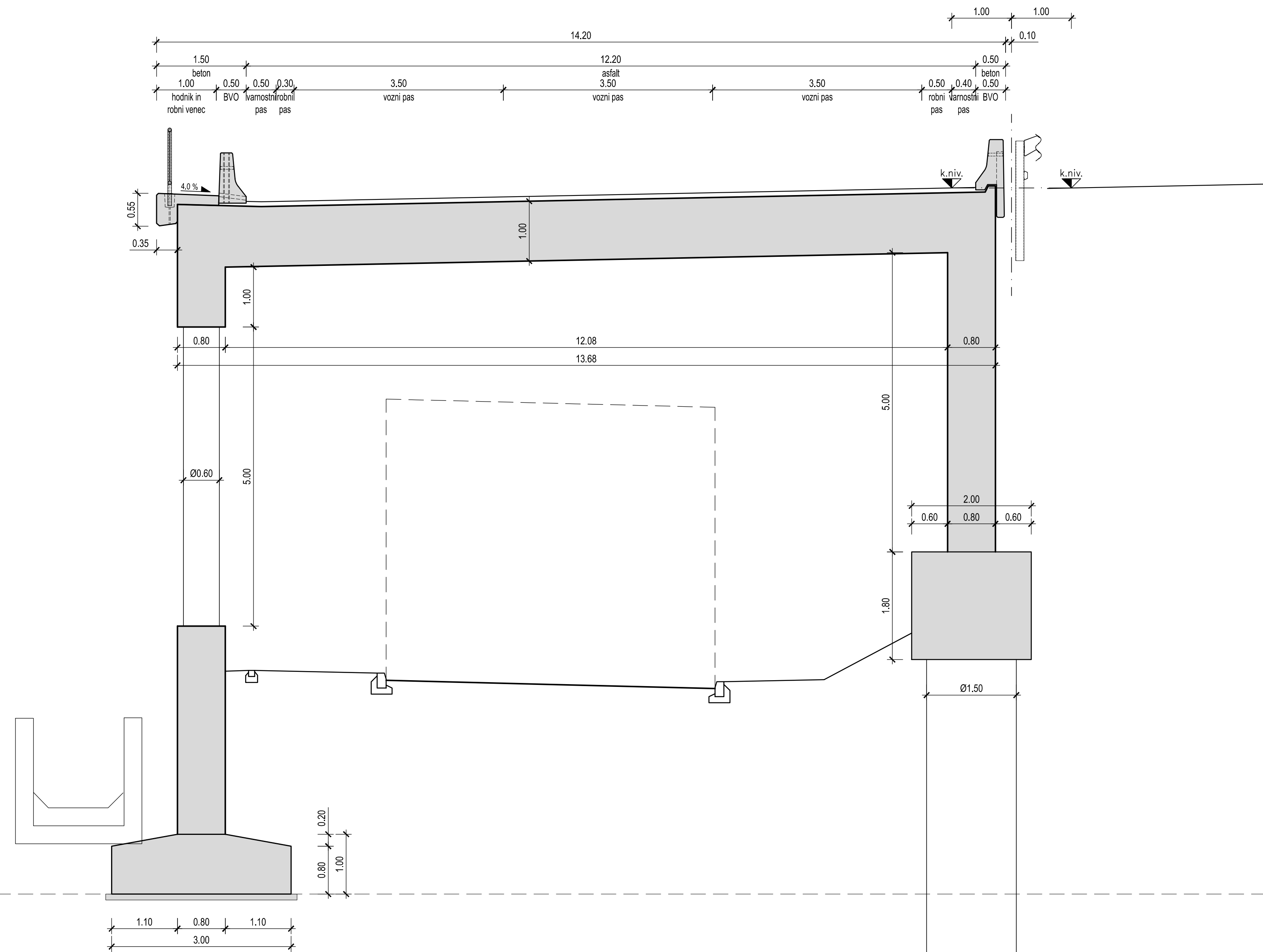
GALERIJA 8-05 PESJE KARAKTERISTIČNA PREČNA PREREZA
