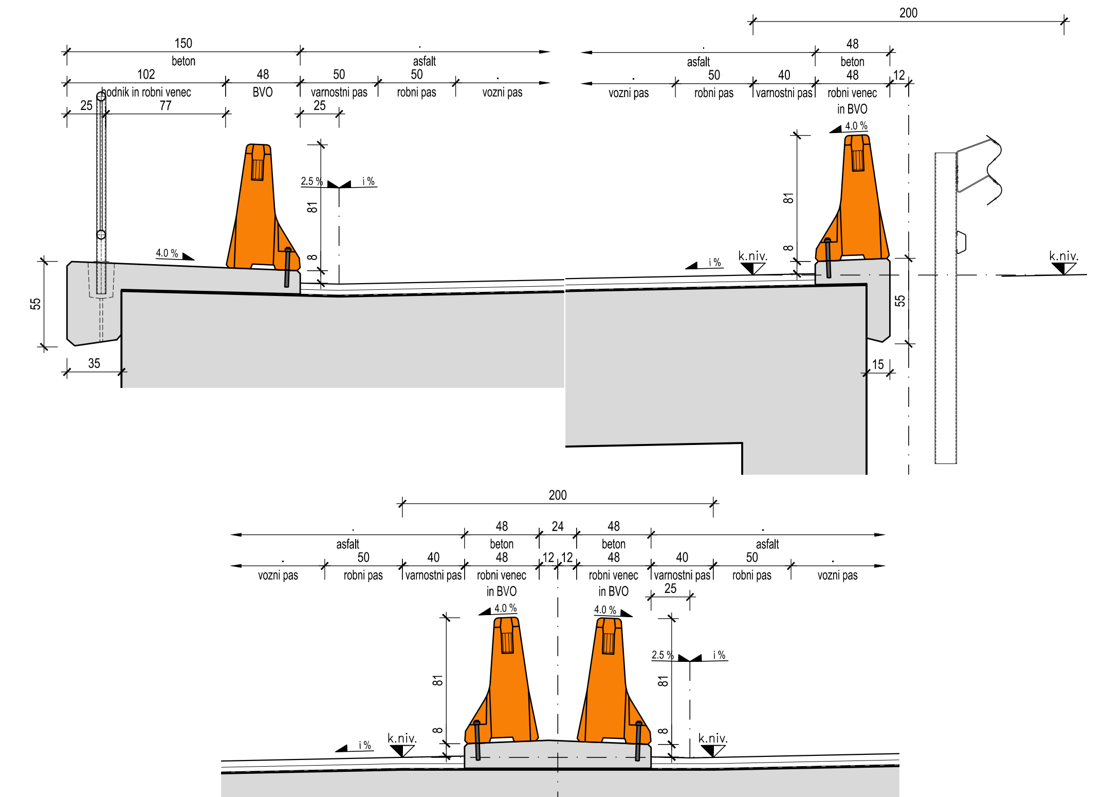
GALERIJA 8-05 PESJE DETAJL H2-W1 merilo 1:25
