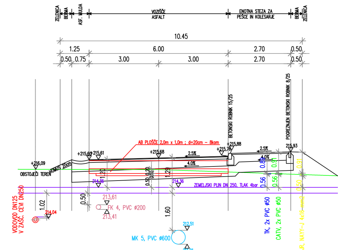
ZNAČILNI PREREZ CESTE JP 804 066 PROFIL PLINOVODA P1
