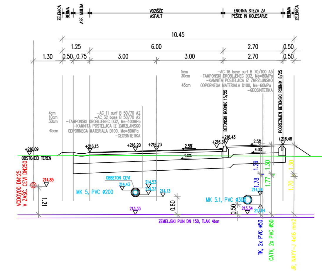
ZNAČILNI PREREZ CESTE LZ 303 011 - PROFIL PLINOVODA P6
