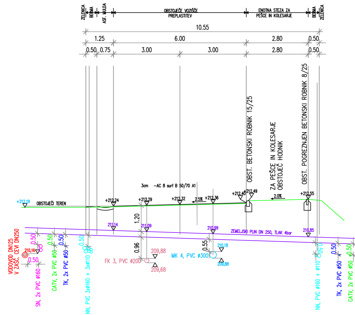
ZNAČILNI PREREZ CESTE LZ 303 011 PROFIL PLINOVODA P5
