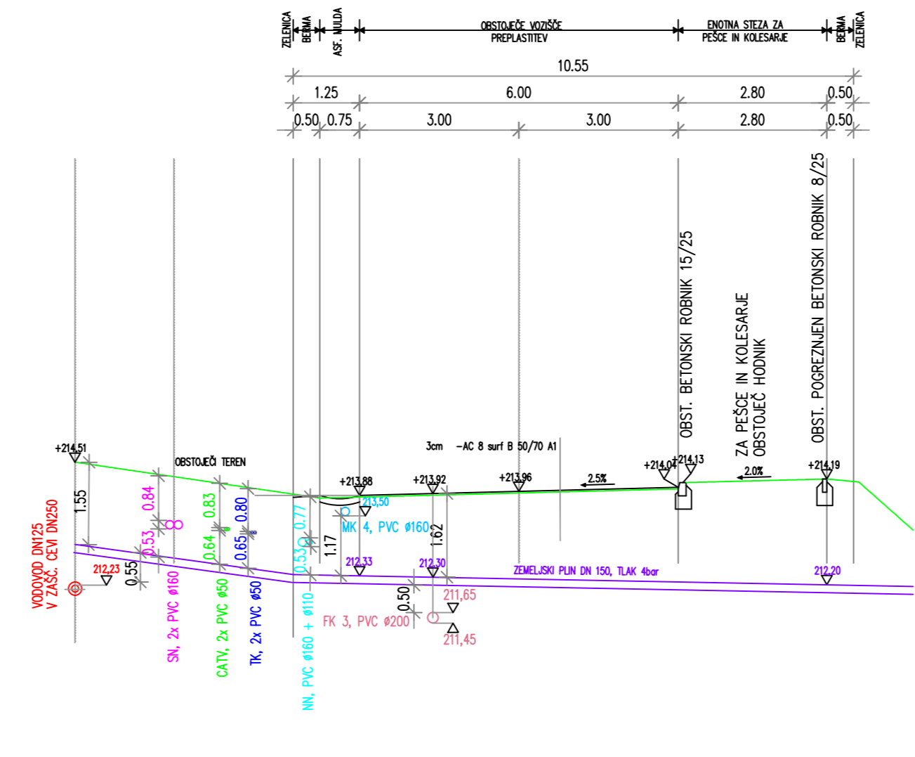
ZNAČILNI PREREZ CESTE LZ 303 011 - PROFIL PLINOVODA P6
