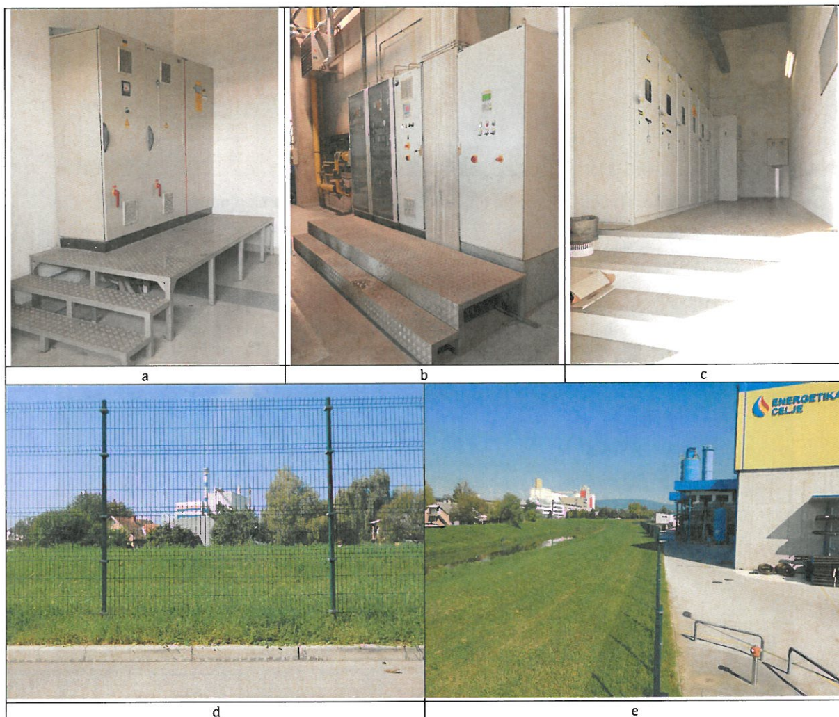
Slika 29: Izvedeni protipoplavni ukrepi na lokaciji Toplarne Celje; dvig vitalne tehnične opreme od tal (slika a,b,c) in izgradnja protipoplavnega nasipa na levem bregu Hudinje (slika d in e) [vir: Toplarna Celje]
