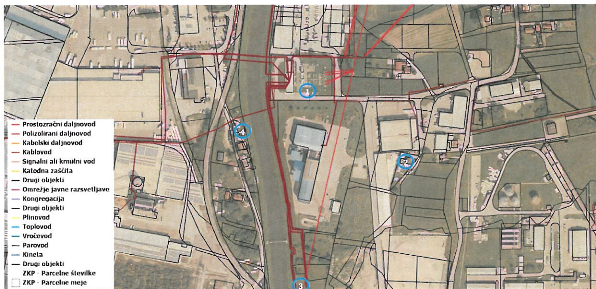
Slika 84: Prostozračni daljnovodi in kablovodi v okolici območja Toplarne Celje
