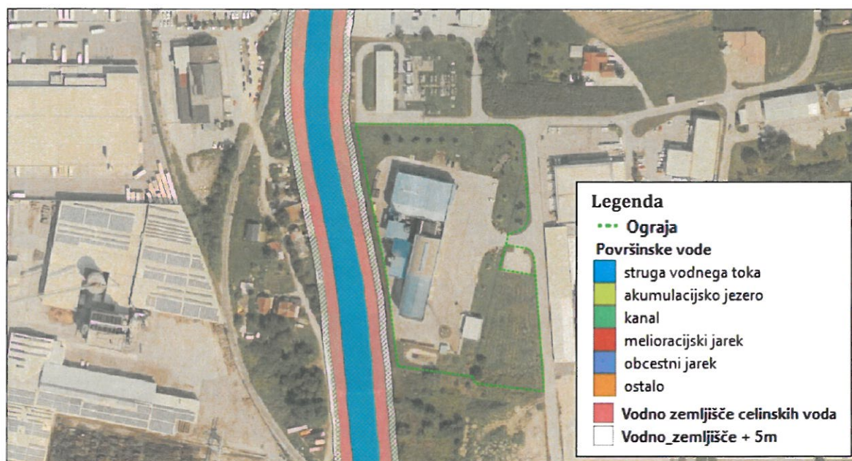
Slika 32: Vodna in priobalna zemljišča v neposredni bližini Toplarne Celje [27]
