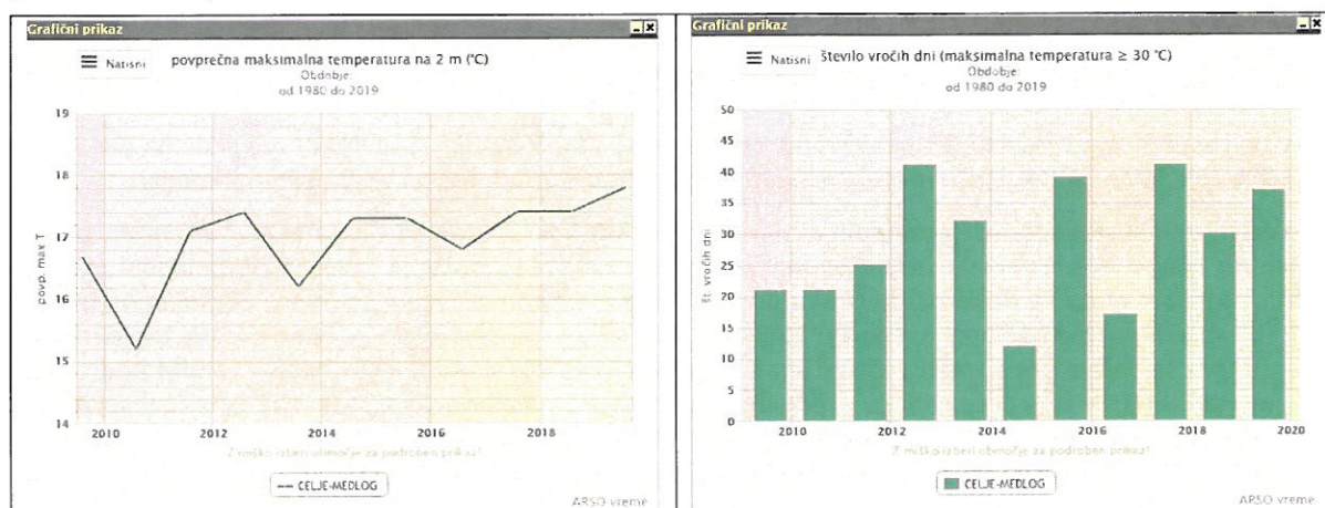
Slika 70: Pregled maksimalne temperature (levo) in števila vročih dni (desno) na merilnem mestu Celje-medlog
