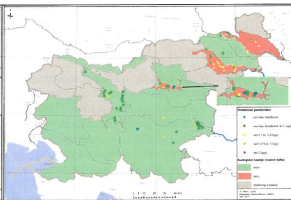
Slika 54: Vsebnost vsote pesticidov v podzemni vodi v letu 2018
