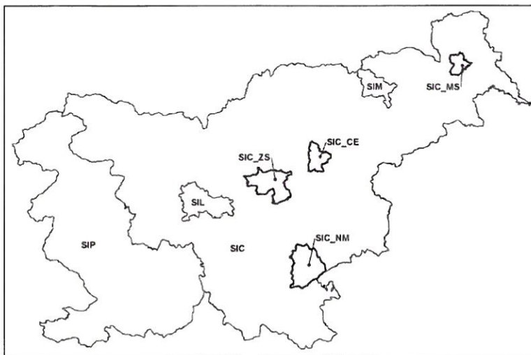
Slika 59: Prikaz območij in podobmočij kot jih določata Odredba [64] in Odlok [65].
