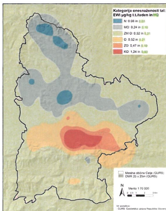
Slika 51: Onesnaženost zgornjega sloja tal s kadmijem na območju Mestne občine Celje [40] in ocenjeni tedenski vnosi (µg/kg t.t./teden) ter koeficient tveganja glede na kategorije onesnaženosti tal
