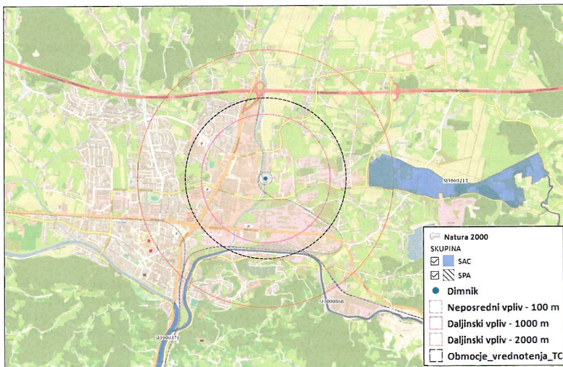
Slika 85: Območja Natura 2000 in zavarovana območja v okolici Toplarne Celje [27]
