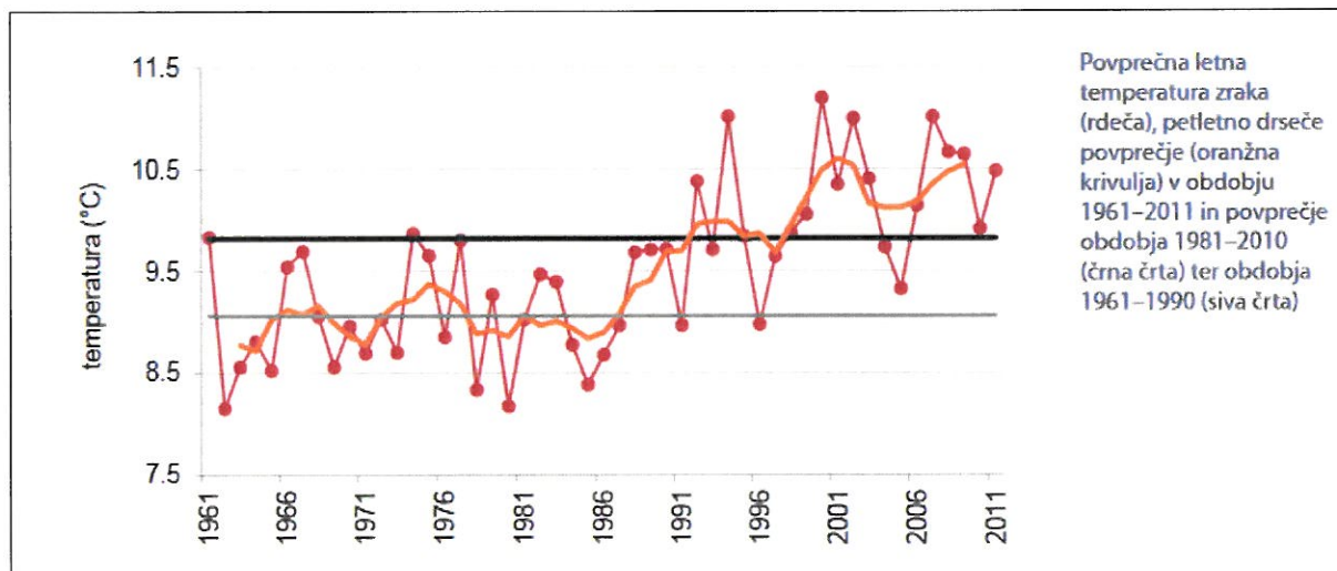
Slika 69: Pregled povprečne temperature na merilnem mestu Celje [73]
