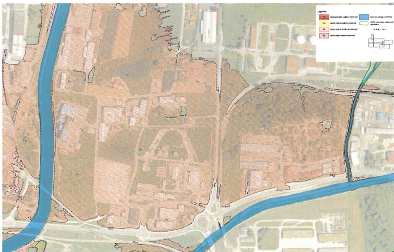
Slika 30: Karta razredov poplavne nevarnosti (Hudinja z V. Ložnico) [24]
