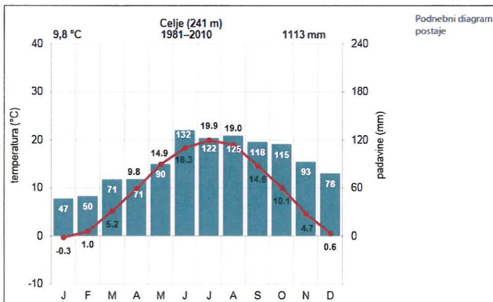
Slika 71: Podnebni diagram merilnega mesta Celje [73]
