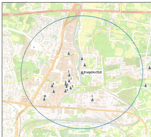
Slika 57: REMIS zavezanci na področju vrednotenja v bližini Energetike Celje.
