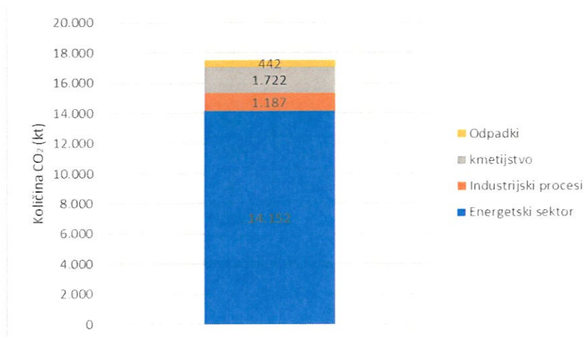
Slika 87: Pregled emisije eq CO 2 po sektorjih
