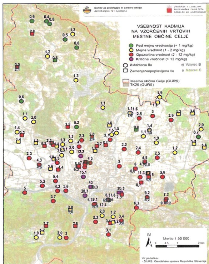
Slika 50: Vsebnost kadmija na vzorčnih vrtovih Mestne občine Celje
