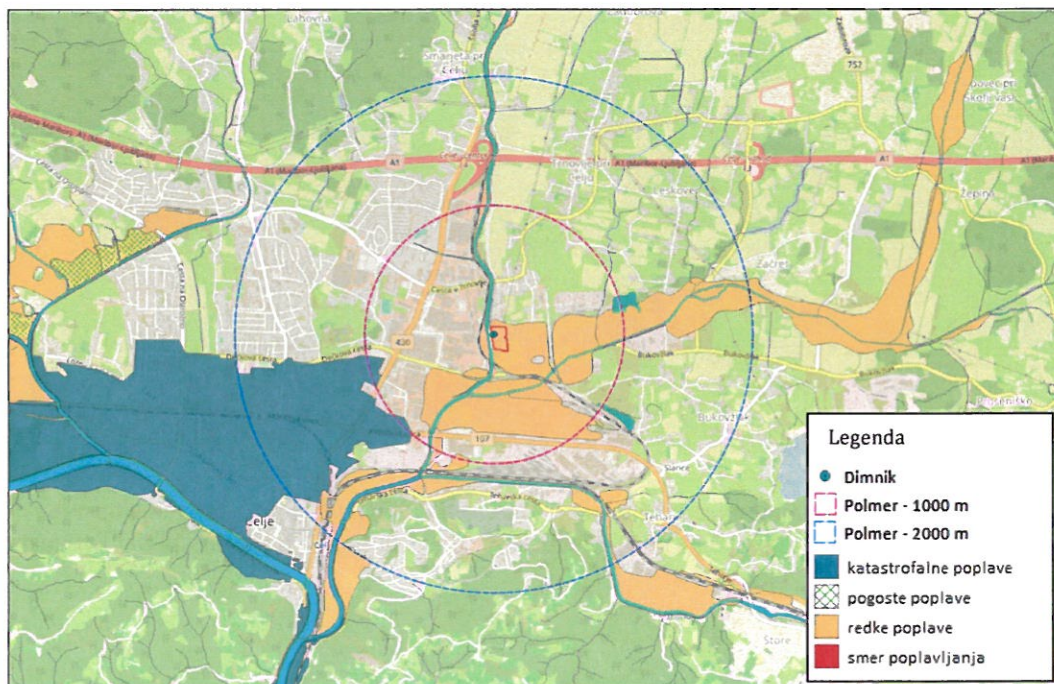
Slika 28: Poplavna območja v okolici Toplarne Celje [27]
