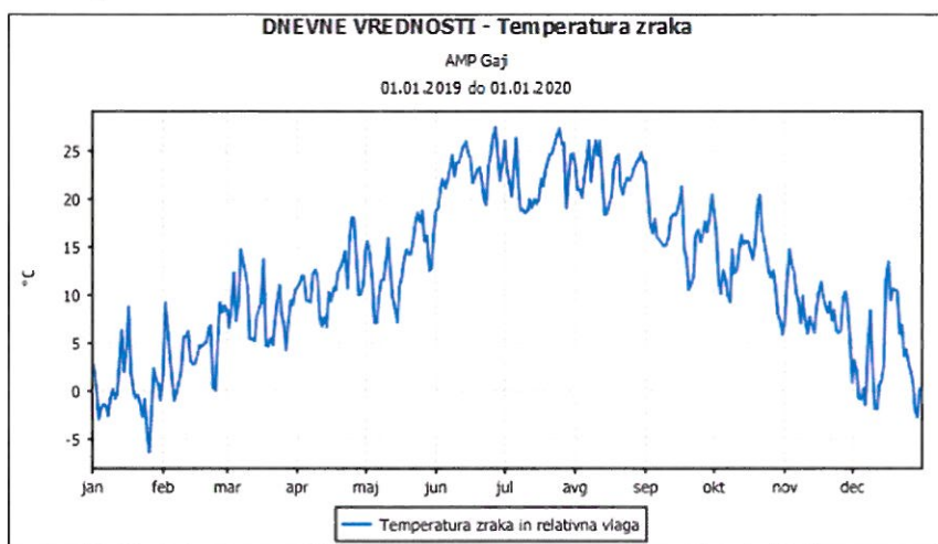
Slika 62: Pregled gibanja temperature zraka v letu 2019.
