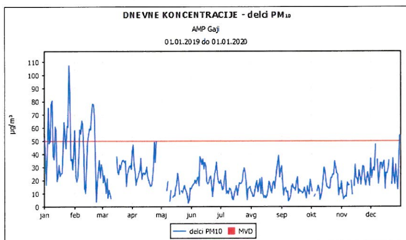
Slika 65: Dnevne koncentracije PM 10 v letu 2019.
