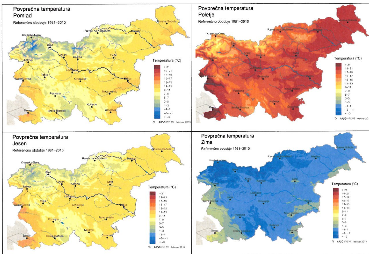
Slika 10: Sezonska povprečna temperatura v referenčnem letu na območju R Slovenije [17]
