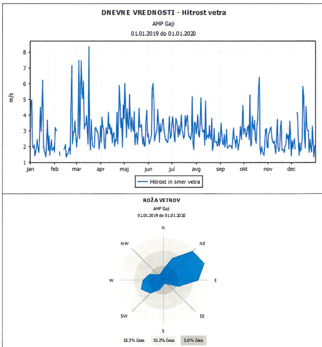
Slika 18: Roža vetrov in hitrost vetra na merilnem mestu Gaji
