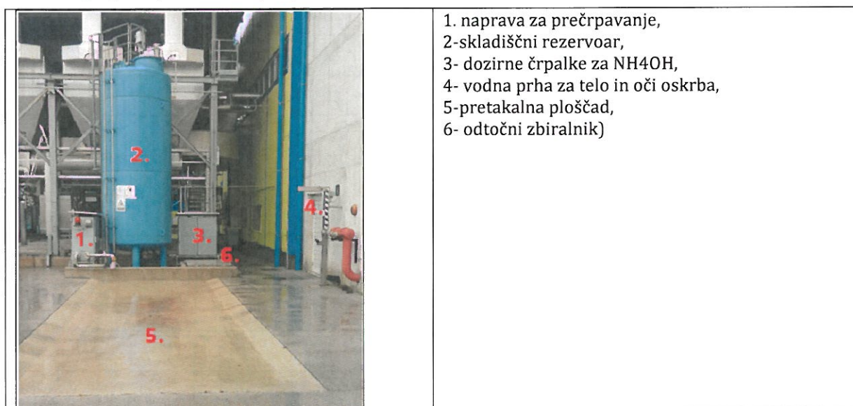
Slika 48: Zunanji del sistema za ravnanje z amonijačno vodo [39]
