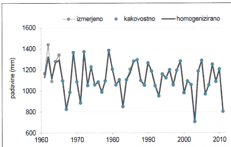
Slika 72: Pregled količine padavin na merilnem mestu Celje [73]
