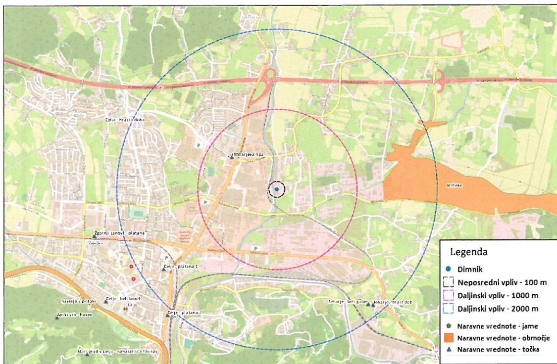
Slika 37: Območja naravnih vrednot v okolici Toplarne Celje [27]
