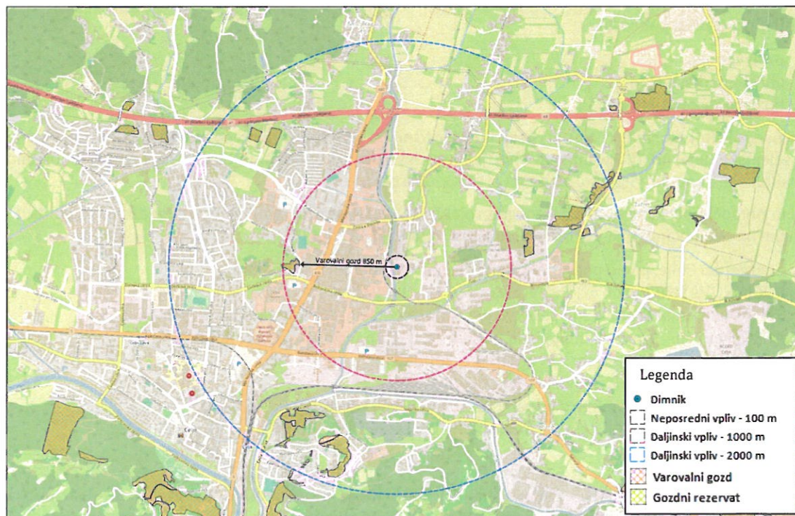
Slika 39: Varovalni gozd in gozdni rezervat v okolici Toplarne Celje [27]
