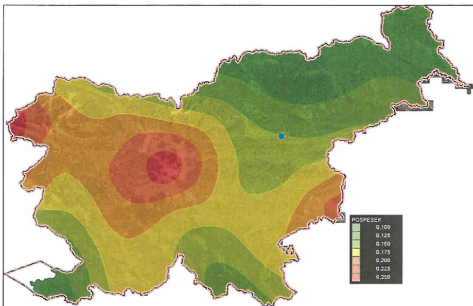
Slika 76: Karta potresne nevarnosti [ARSO]
