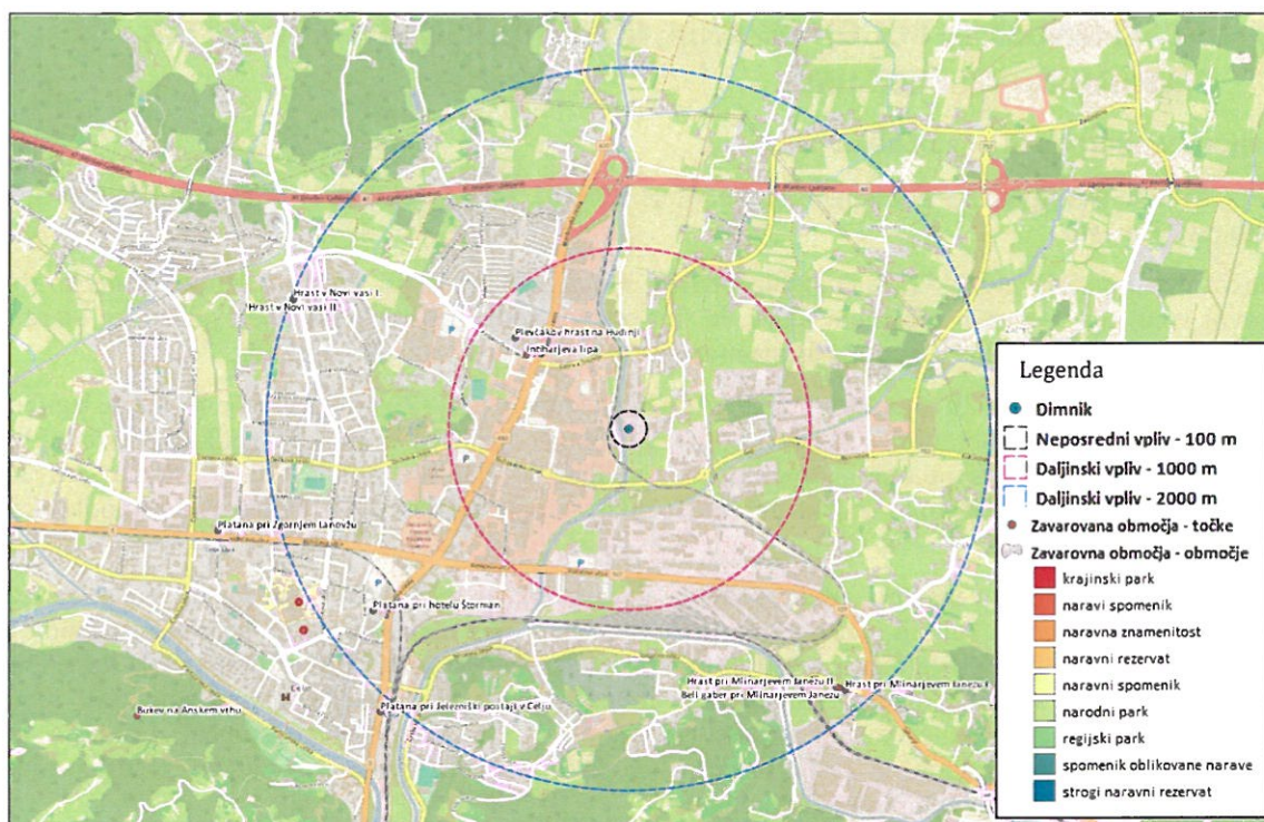
Slika 38: Zavarovana območja v okolici Toplarne Celje [27]
