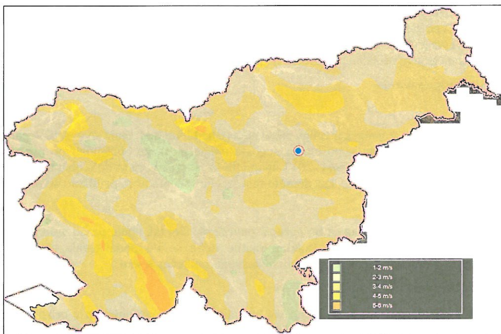
Slika 75: Povprečna letna hitrost vetra 10 m nad tlemi model DADA (obdobje 1994–2001) [ARSO]
