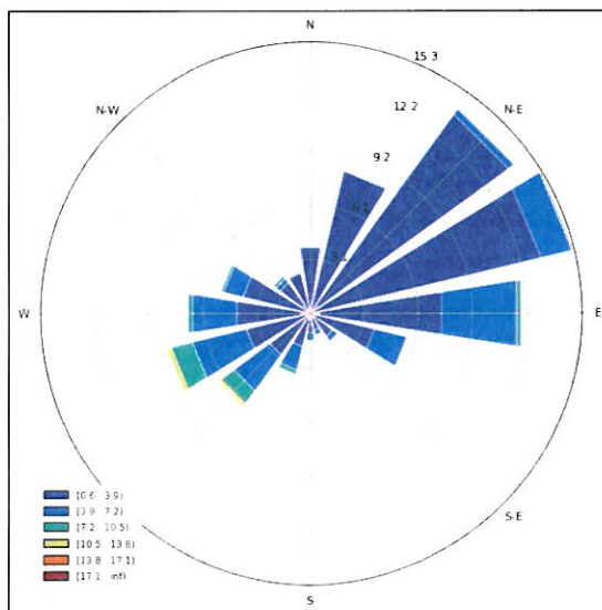
Slika 61: Roža vetrov na lokaciji Gaji.
