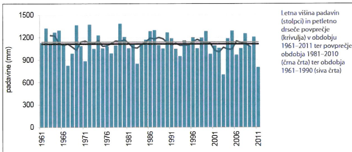
Slika 73: Letna višina padavin z oznako višine padavin v referenčnih letih na merilnem mestu Celje [73]
