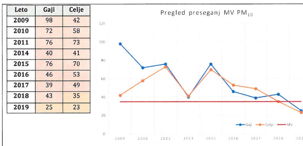
Slika 68: Število preseganj dnevne mejne vrednosti po posameznih letih na merilnem mestu Gaji in Celje
