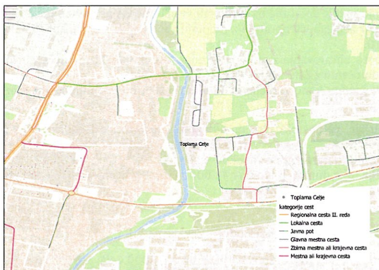
Slika 86: Prikaz kategorije cest na območju obravnavanega objekta.
