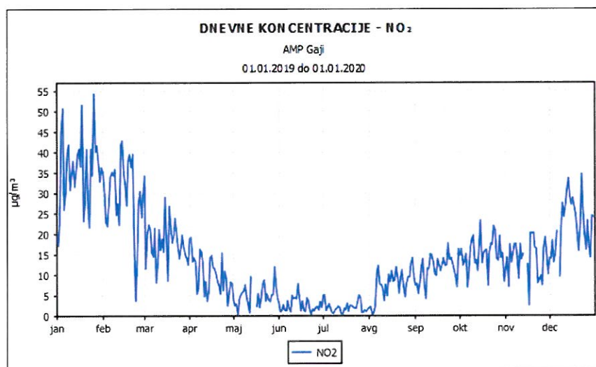
Slika 64: Dnevne koncentracije NO 2 v letu 2019.
