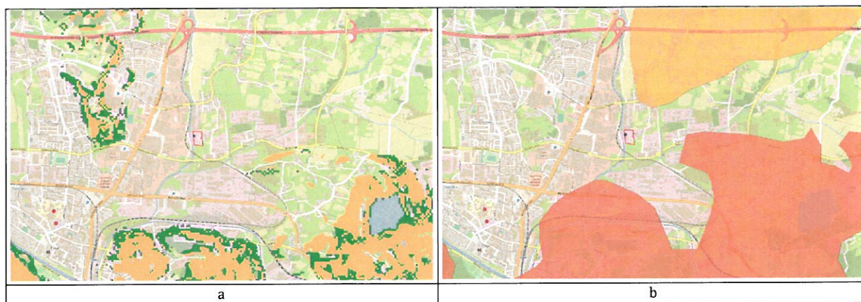
Slika 34: Plazljiva območja (a) in erozijska območja (b) v okolici Toplarne Celje [27]
