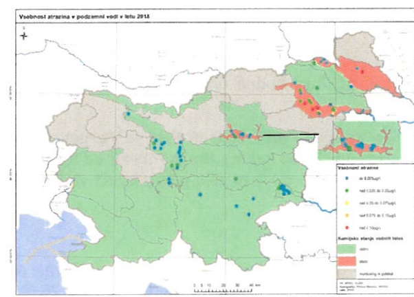
Slika 55: Vsebnost atrazina v podzemni vodi v letu 2018
