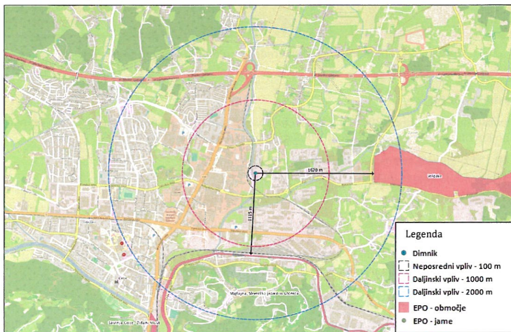
Slika 36: Ekološko pomembno območje v okolici Toplarne Celje [27]
