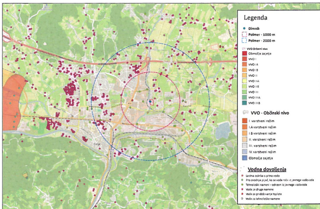
Slika 27: Vodovarstvena območja ter izdana vodna dovoljenja na območju Celja [27]
