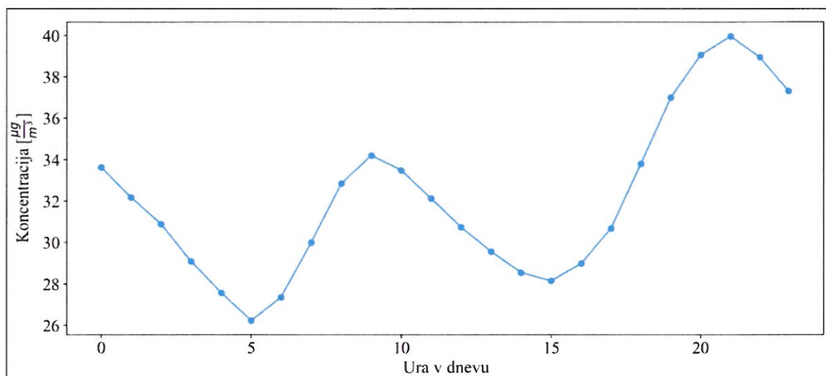
Slika 67: Dnevni hod koncentracij PM 10
