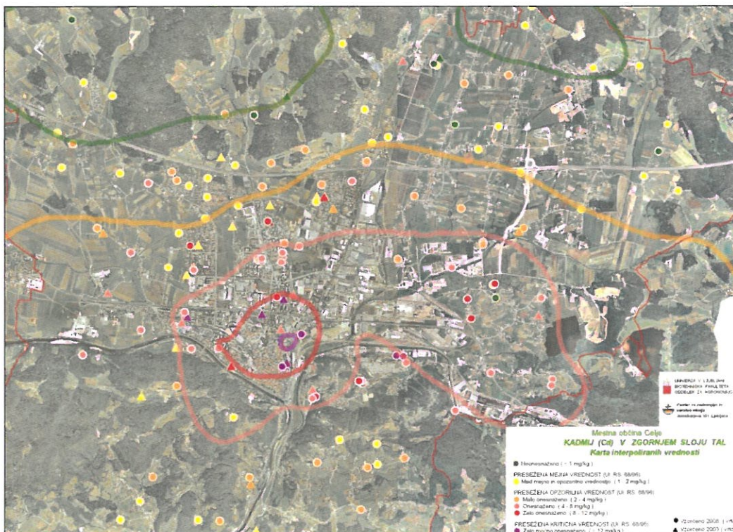
Slika 52: Koncentracija kadmija v zgornjem sloju tal v Mestni občini Celje
