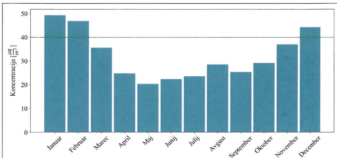
Slika 66: Povprečne mesečne koncentracije PM 10
