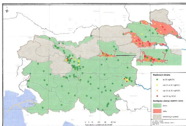
Slika 53: Vsebnost nitrata v podzemni vodi v letu 2018
