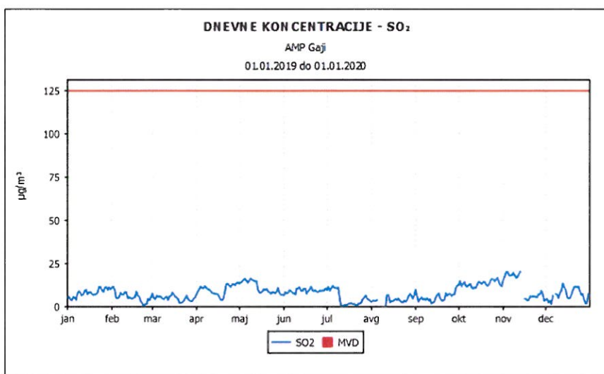
Slika 63: Dnevne koncentracije \text{SO}_2 v letu 2019.
