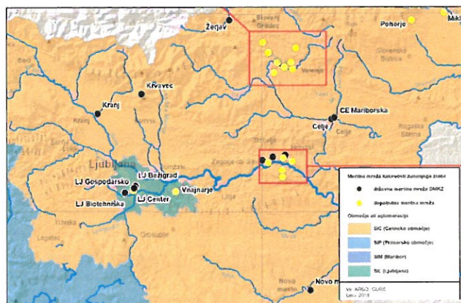
Slika 58: Merilna mreža kakovosti zunanjega zraka [63]
