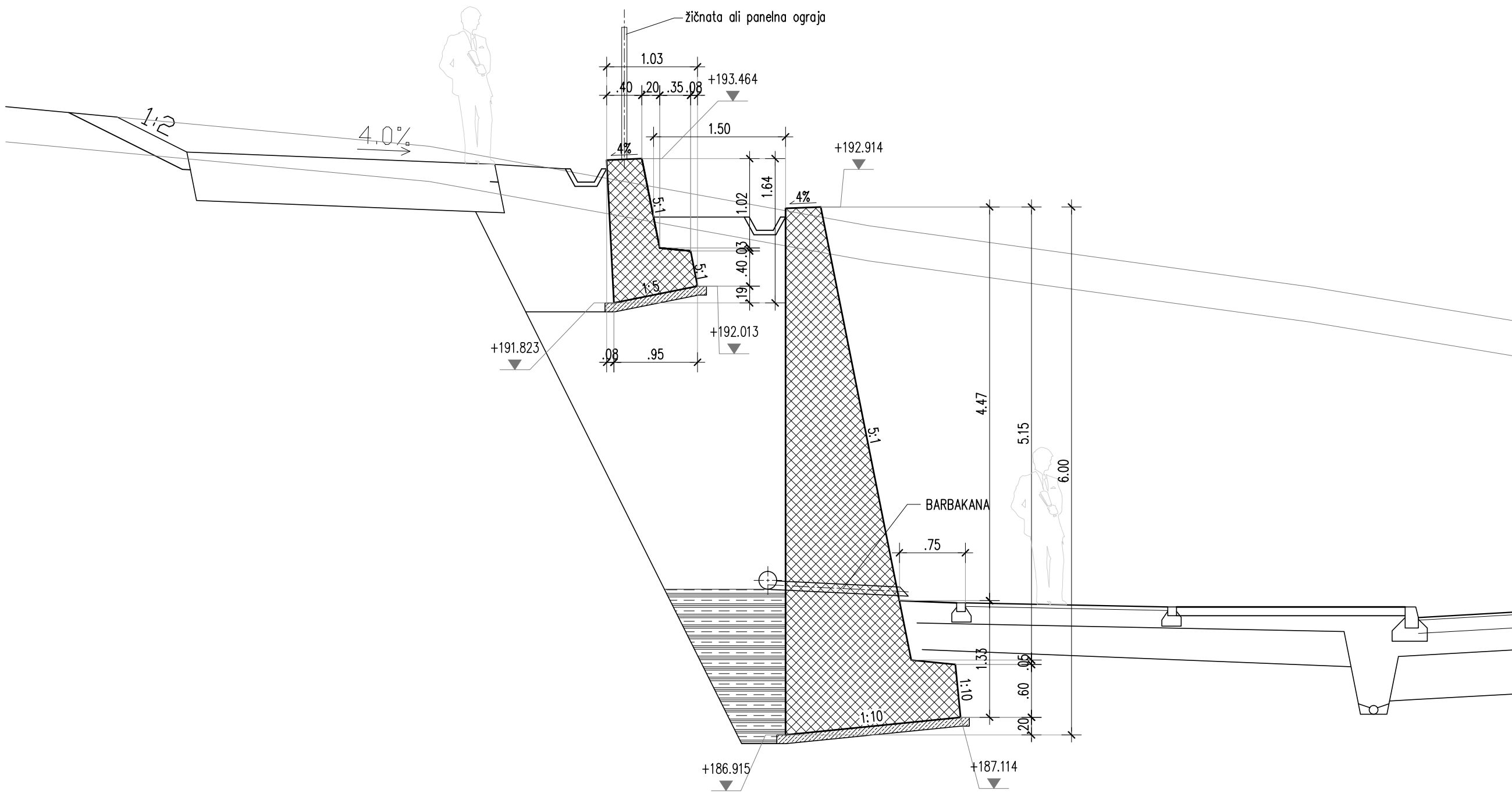
KARAKTERISTIČNI PREČNI PREREZ - P24 M 1:50
