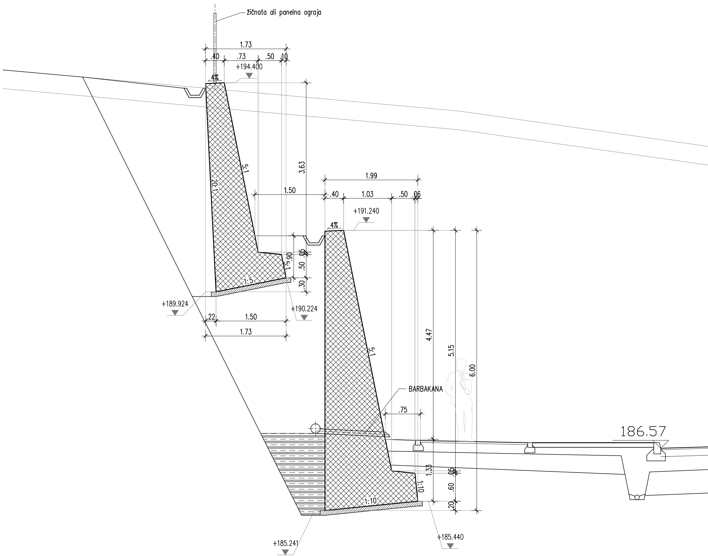
KARAKTERISTIČNI PREČNI PREREZ - P25 M 1:50
