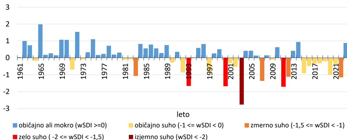
Slika 3.7: Letni (zgoraj) in polletni (spodaj) sušni indeks pretoka za Slovenijo v obdobju 1961–2023; polletni sušni indeks velja za obdobje od aprila do septembra
