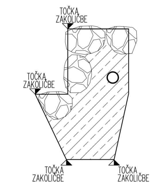
OK-1, OK-2, OK-3 Podest iz lomljenca v betonu za podbetoniranje obal. zidov
