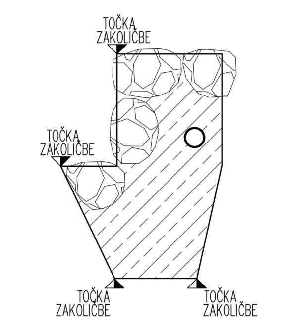
OK-1, OK-2, OK-3 Podest iz kamnjaca v betonu za podbetoniranje obst. židov
