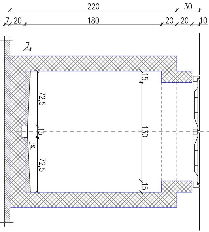
PREREZ A-A
