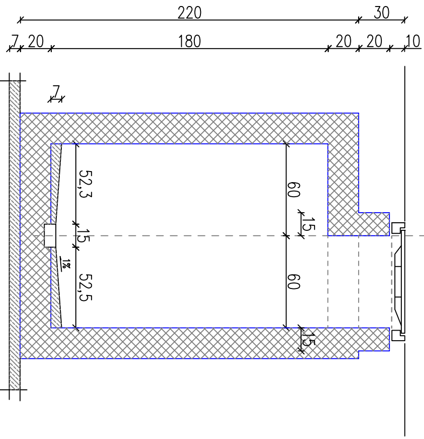
PREREZ B-B
