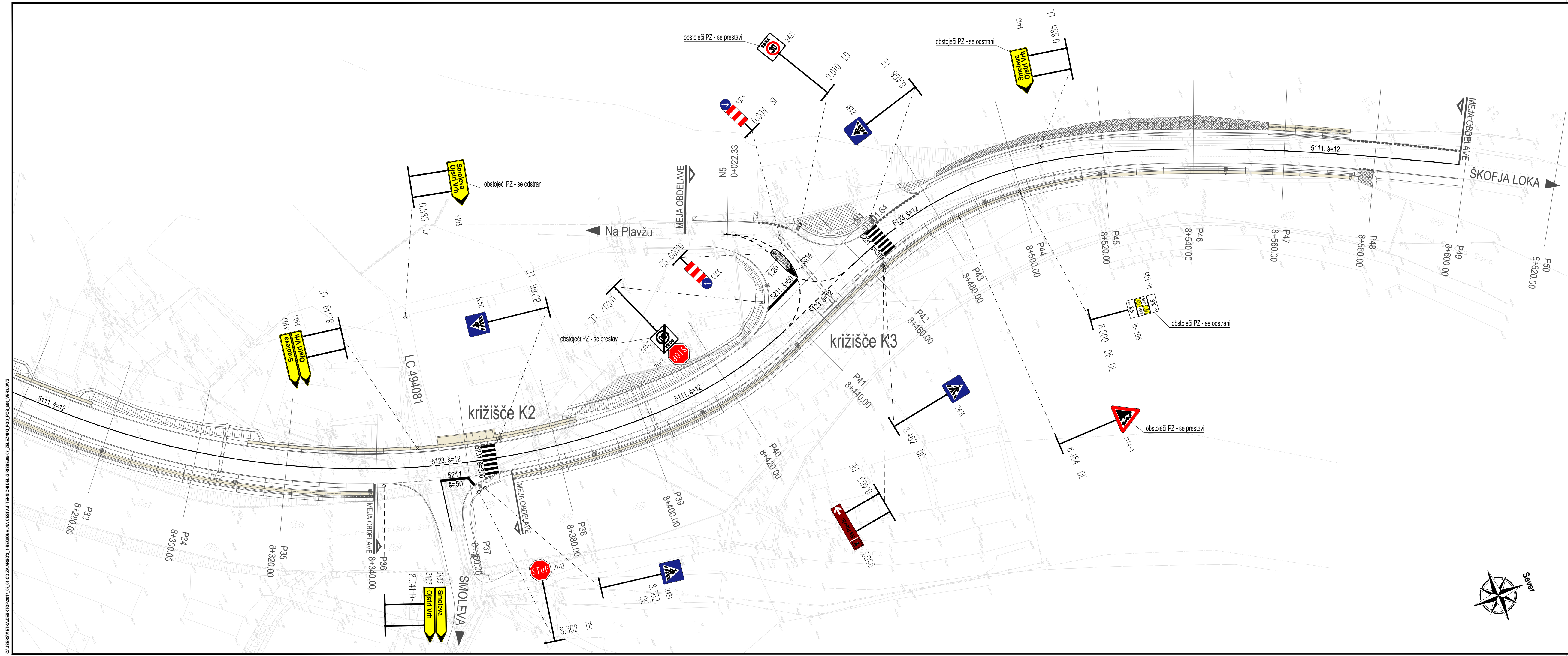
Situacija prometne ureditve od km 8+240 do km 8+599 M 1:500
