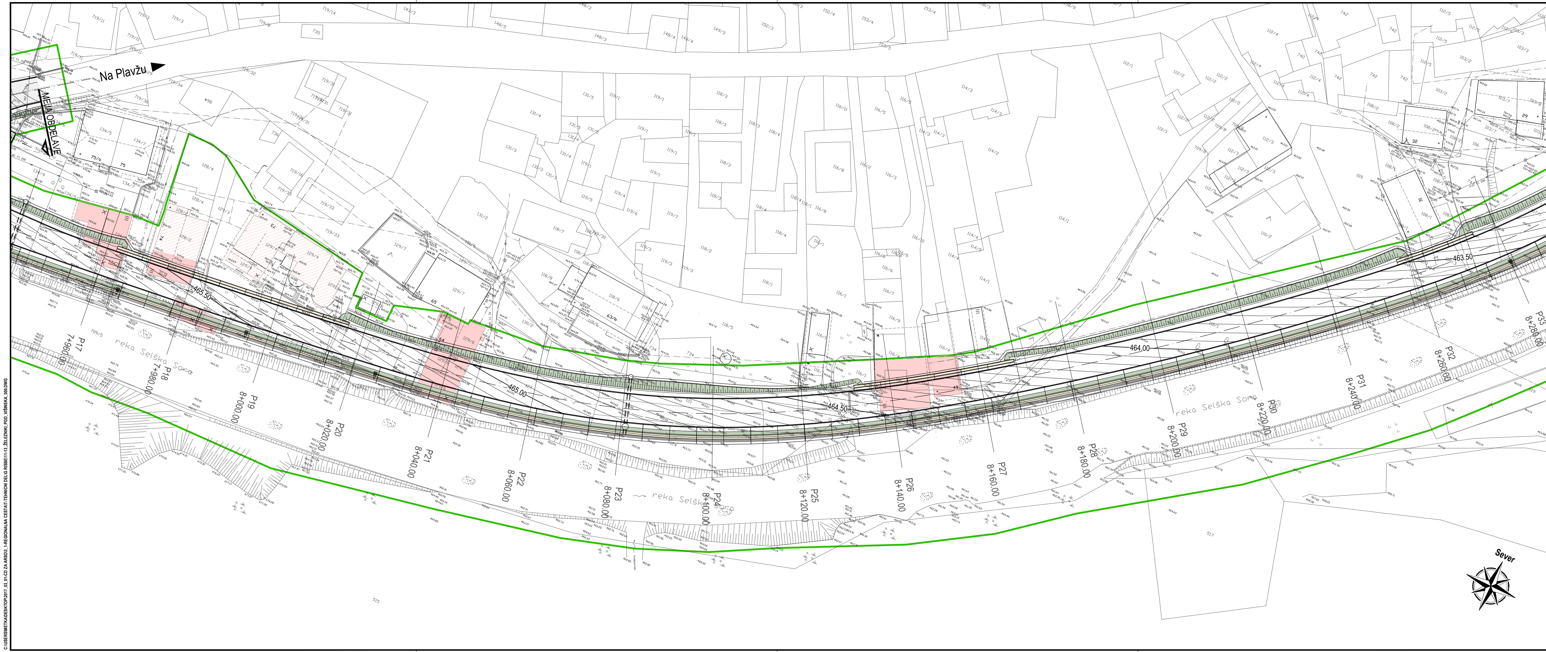
Višinska situacija od km 7+920 do km 8+240 M 1:500
