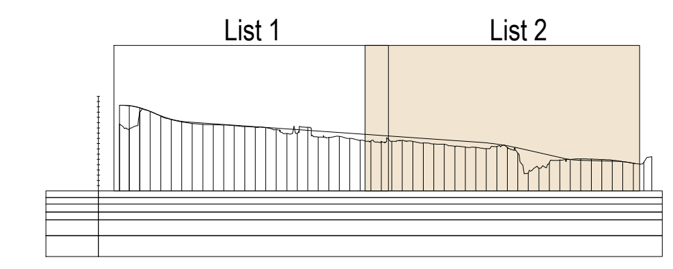
Vzdolžni profil Regionalna cesta List 2/2 M 1:1000/100
