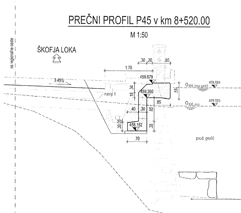
Slika 1: Geometrija zidu
