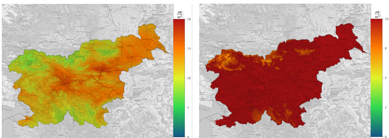
Slika 4.4: Prostorska porazdelitev modelske ocene povprečne letne vrednosti delcev \text{PM}_{2,5} v letu 2024 glede na AQ direktivo iz leta 2008 (levo) in revidirano AQ direktivo (desno). Rezultati modela CAMx so naknadno izboljšani z data fusion procesom z upoštevanjem nadmorske višine in naknadno vključitvijo meritev.
