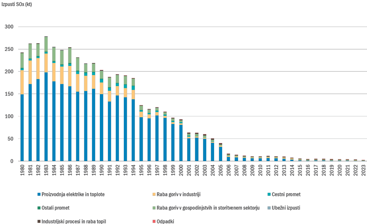
Slika 11.1: Letni izpusti \text{SO}_x po virih v Sloveniji
