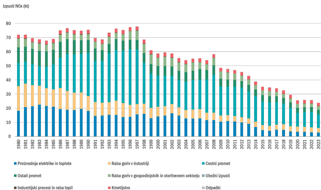
Slika 10.1: Letni izpusti dušikovih oksidov po sektorjih v Sloveniji
