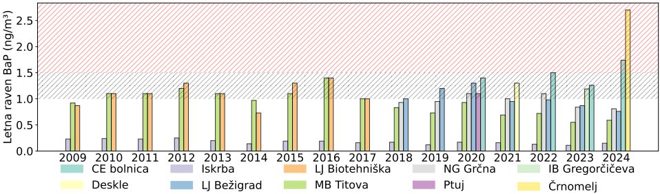
Slika 8.2: Prikaz povprečnih letnih ravni benzo(a)pirena na različnih postajah po letih. Ciljna vrednost je 1 \text{ ng}/\text{m}^3 .
