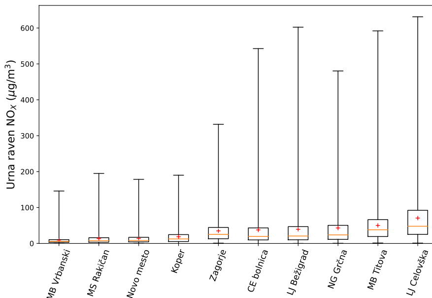
Slika 10.6: Urne ravni \text{NO}_x na merilnih mestih DMKZ v letu 2024. Prikazane so najnižja in najvišja izmerjena raven (spodnja in zgornja vodoravna črta), oba kvartila (vrh in dno pravokotnika) in mediana (oranžna vodoravna črta v pravokotniku). Znak + označuje letno raven.
