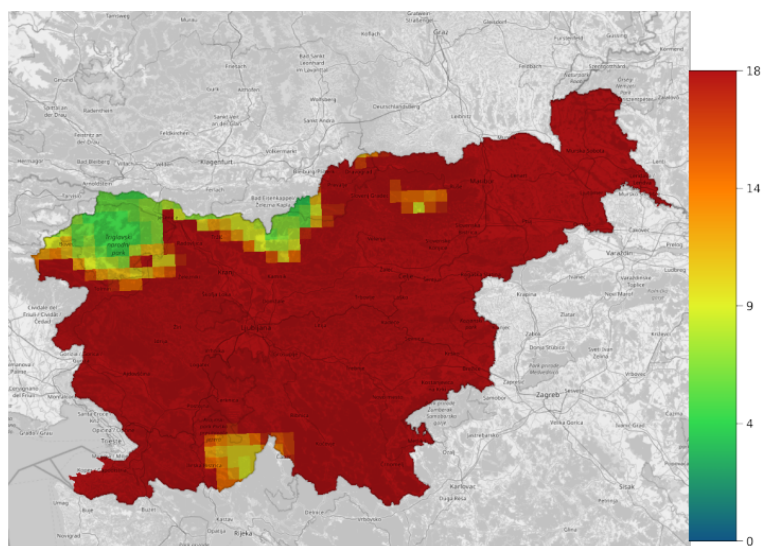
Slika 4.3: Prostorska porazdelitev modelske ocene števila preseganj mejne dnevne vrednosti delcev \text{PM}_{2,5} ( 25 \mu\text{g}/\text{m}^3 ) v letu 2024 glede na revidirano AQ direktivo.
