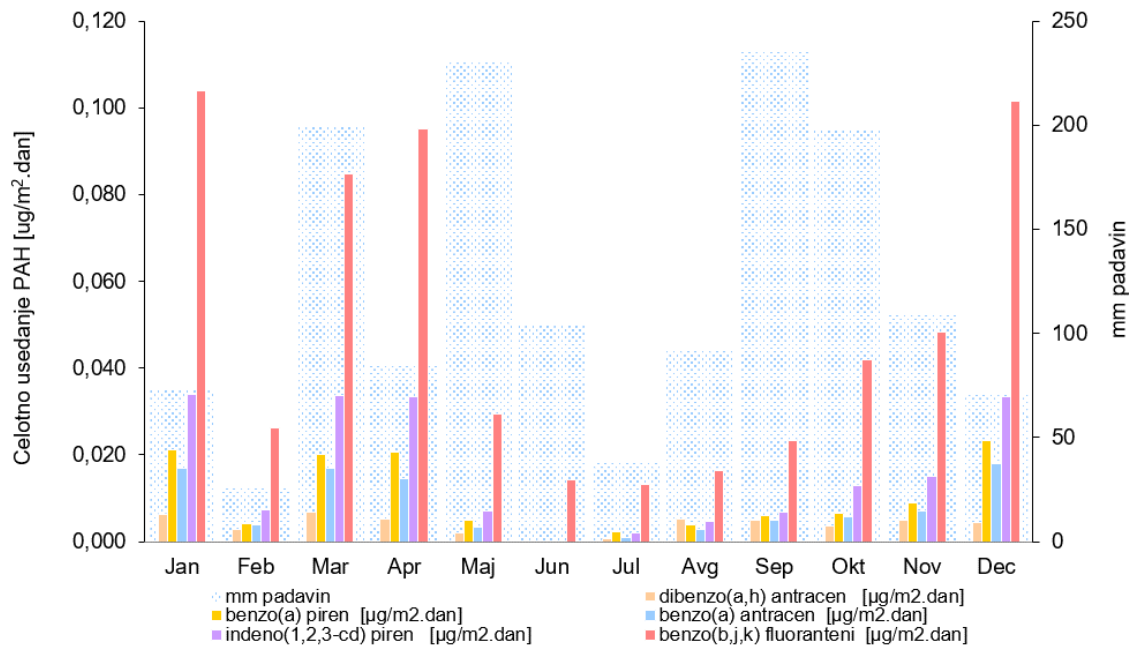
Slika 15.22: Celotno usedanje nekaterih PAH po mesecih v letu 2024 µg/m²dan
