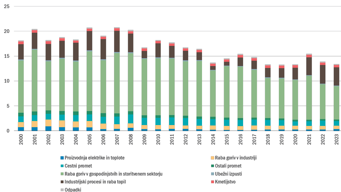
Izpusti PM 10 (kt)
