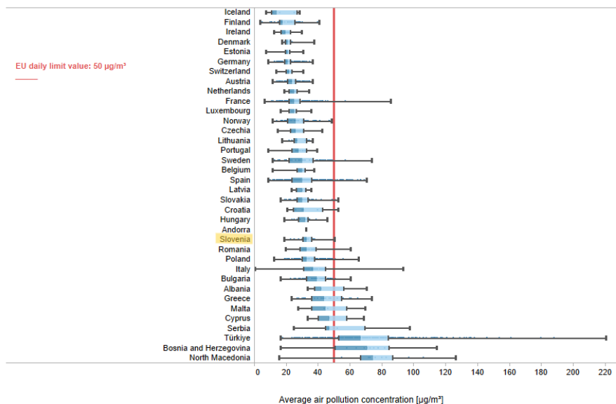
Slika 3.2: Primerjava dnevnih ravni PM_{10} (90,4. percentil oz. 36. najvišja vrednost) v letu 2023 na vseh poročanih merilnih mestih po državah z mejno dnevno vrednostjo EU (rdeča črta). Za vsako državo so prikazani minimum, maksimum, mediana ter 25. in 75. percentil.
